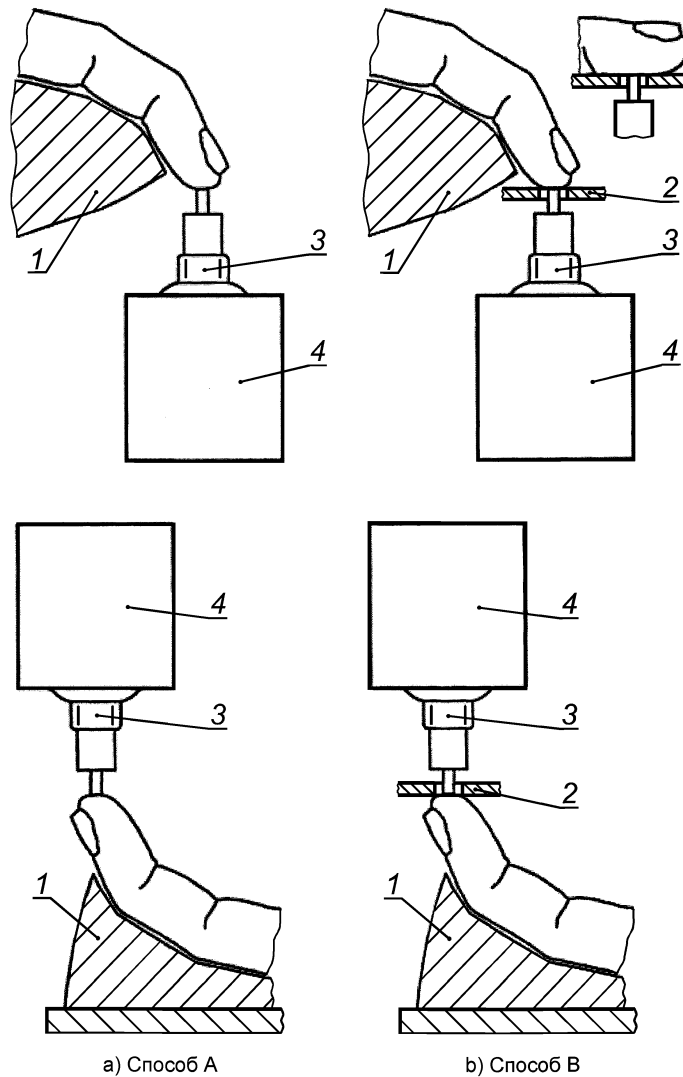
1 — опора пальца; 2 — подставка; 3 — датчик; 4 — стимулятор
