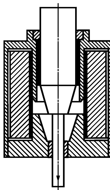
Рисунок А.3 — Поперечный разрез соленоида
