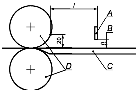
Рисунок 101 — Размеры загрузочного отверстия катковых гладильных машин
