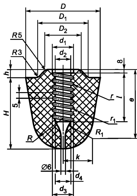
Рисунок 2 — Стопорная пробка номеров 9—14
