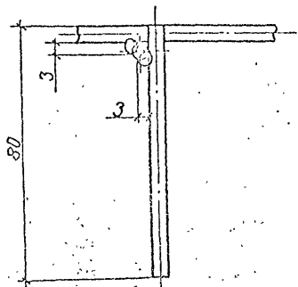
A-A (1:1)
