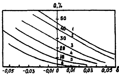
Рис. 2.2. Зависимость относительного количества жидкости Q , перелившейся через обвалование, от параметра b , характеризующего наклон подстилающей поверхности, при различных отношениях a/h_0 :
