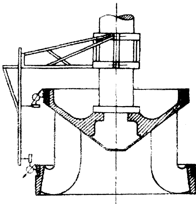
Рис.2. Приспособление для проверки концентричности
