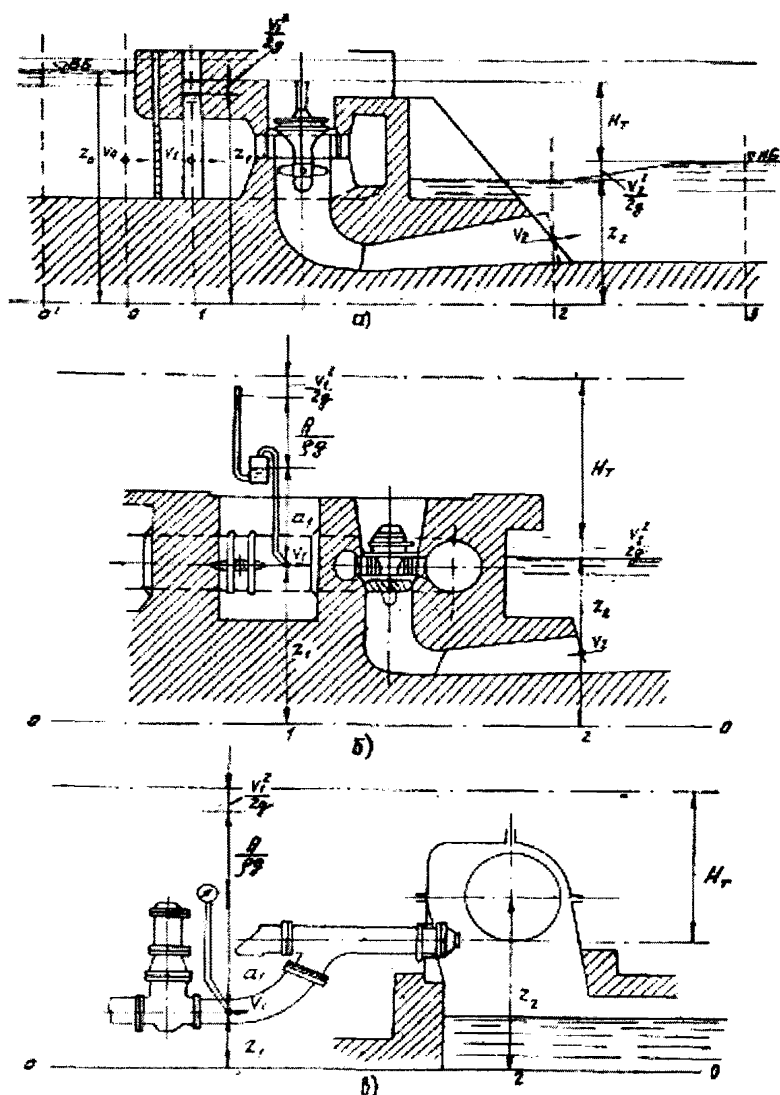
Рис.2. Схема определения напора: а - для низконапорной реактивной турбины; б - для высоконапорной реактивной турбины; в - для ковшовой турбины
