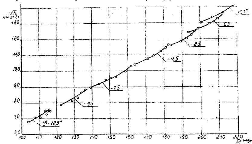
Рис. 24. Пропеллерные расходящие характеристики
