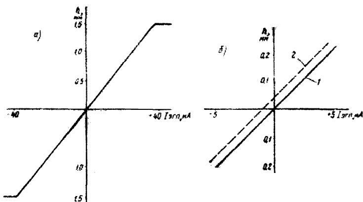
Рис. 11. Статическая характеристика ЭГП.
