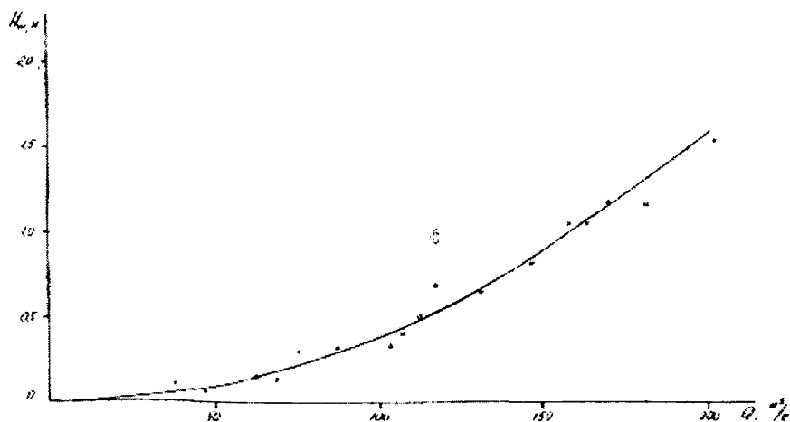
Рис.16. График зависимости потерь напора в турбинном водоводе от расхода воды
