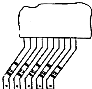
РИС.-2 СХЕМА УСТАНОВКИ ТЕРМОПАР (ТП) И ТЕРМОСТАТИЧЕСКИХ (ТЗ) НА ЛОБОВЫХ ЧАСТЯХ ОБМОТКИ СТАТОРА ГИДРОГЕНЕРАТОРА.
