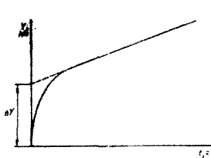
Рис.2. Переходная характеристика открытого направляющего аппарата
