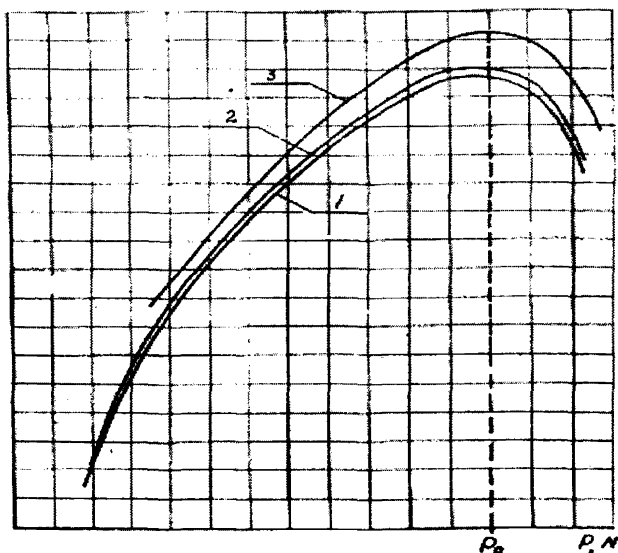
Рис.19. Рабочие характеристики гидротурбинного блока (1), гидроагрегата (2) и гидротурбины (3)
