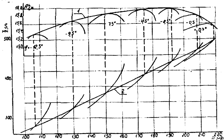
Рис. 25. График для определения координат оптимальной комбинаторной зависимости
