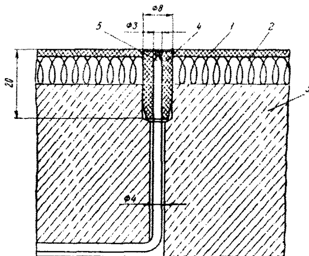
Рис.5. Установка термопары на поверхности ЭМИ-сегмента: 1 - слой чистого фторопласта; 2 - бронзовые проволочные спирали; 3 - стальное основание сегмента; 4 - фторопластовая втулка; 5 - термопара, установленная в отверстие и уплотненная втулкой
