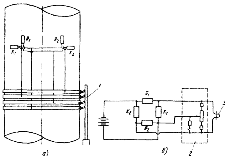
Рис.1. Схемы измерения осевого усилия на валу:
