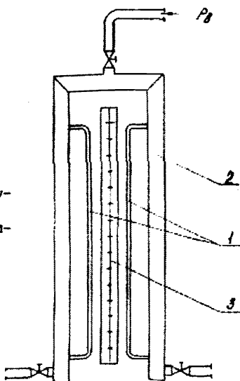
Рис.6. Чашечный дифманометр
