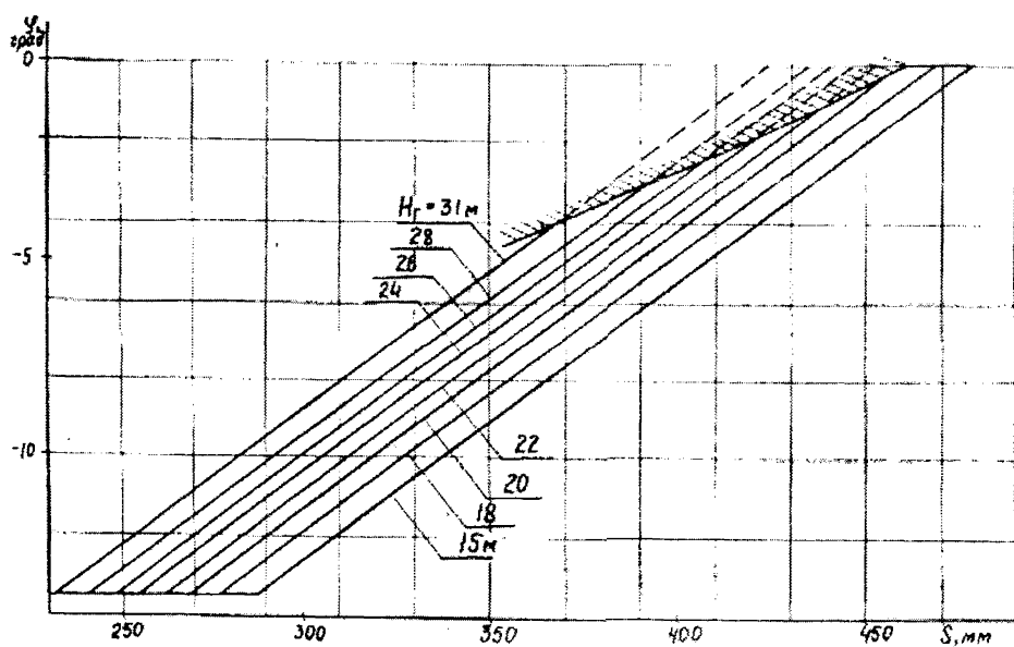
Рис. 27. Оптимальные комбинаторные зависимости для рабочего диапазона напоров
