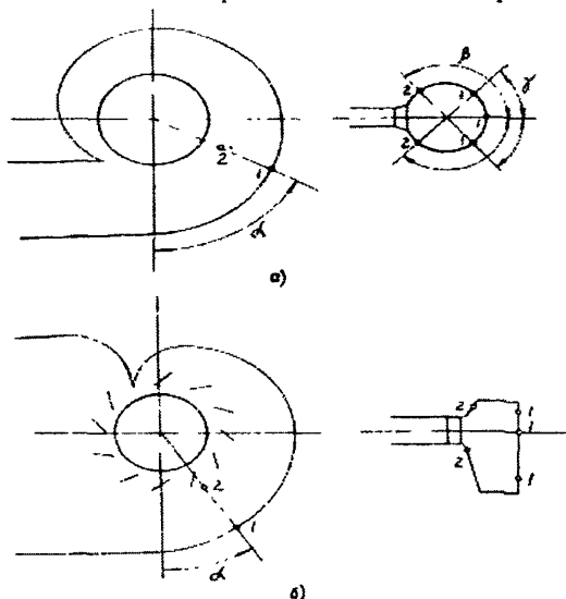
Рис.1. Схема расположения пьезометрических выводов 1 и 2: \alpha - в металлической спиральной камере ( \alpha = 45-90^\circ ; \beta = \pm 30^\circ ; \gamma = 0 \pm 45^\circ ); \delta - в бетонной спиральной камере ( \alpha = 20-60^\circ )
