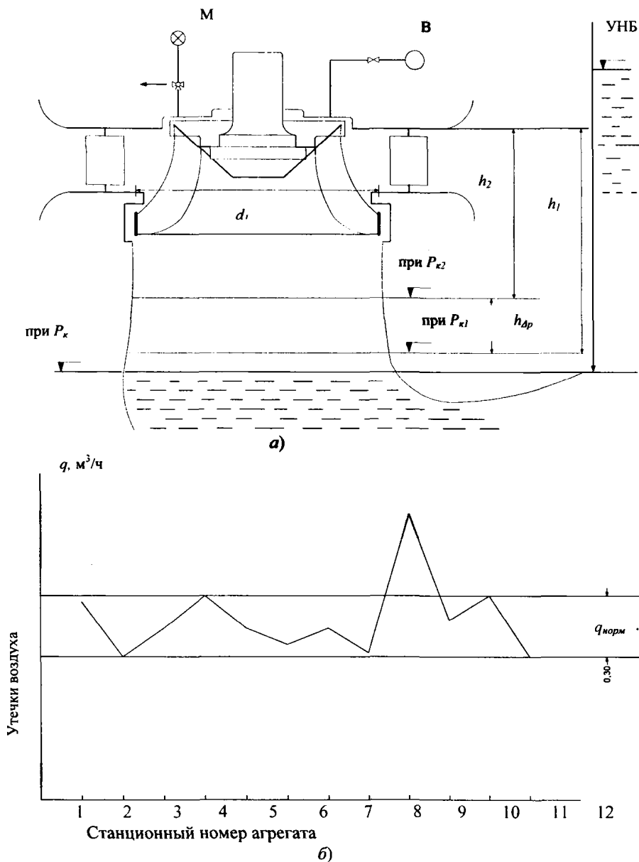
Рис.1. Контроль утечки воздуха из камеры рабочего колеса турбины при работе в режиме СК: а — схема ; б — кривая изменения утечки воздуха из камеры рабочего колеса турбины
