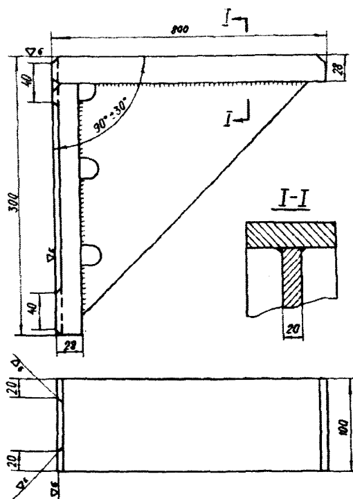
Рис.6. Уголок для проверки диаметров валов с помощью уровня
