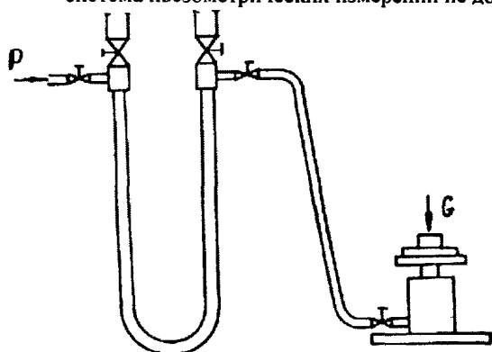
Рис.3. Схема соединения грузопоршневого манометра с дифманометром
