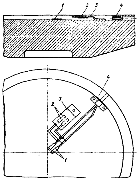
Рис.2. Расположение тензометров на опорной тарелке:
