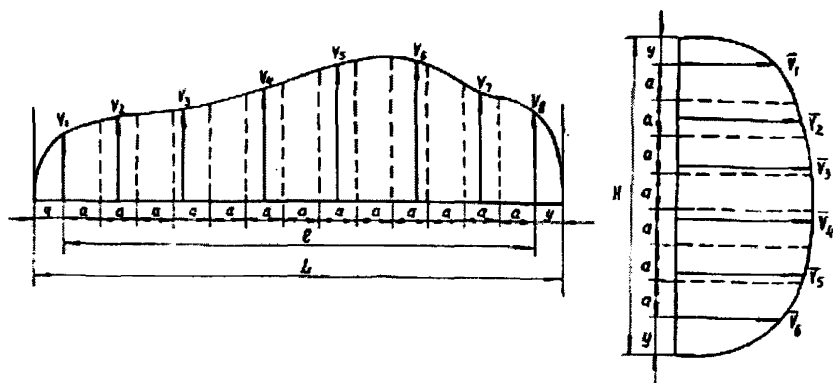
Рис.13. Эпюры скоростей в мерном створе прямоугольного сечения
