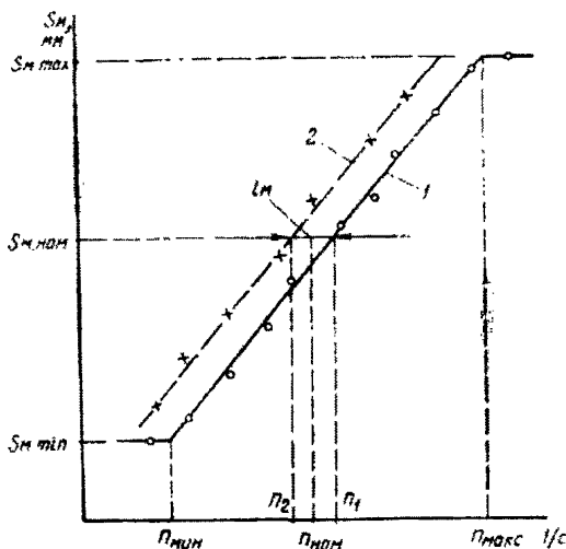
Рис. 1. Статическая характеристика маляка с зоной нечувствительности:
