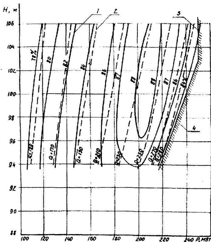
Рис.2I. Эксплуатационная характеристика гидротурбинного блока: 1 - линии равных КПД; 2 - линии равных расходов; 3 - линия ограничения мощности генератора; 4 - линия ограничения мощности турбины
