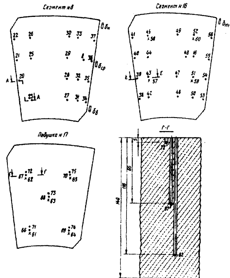
Рис.4. Расположение точек измерения температуры подпятника агрегата № 6 ДДГЭС:
