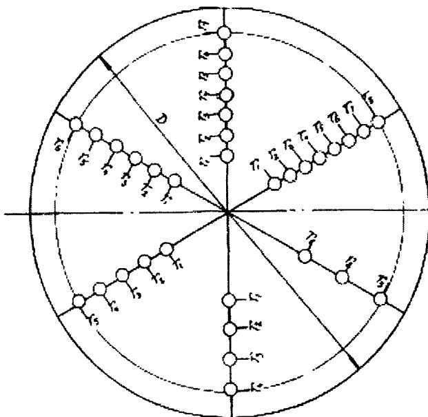
Рис.10. Схема расположения вертушек в круглом трубопроводе
