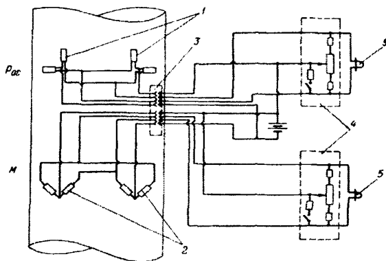
Рис.7. Электрическая схема измерений при определении коэффициента трения:
