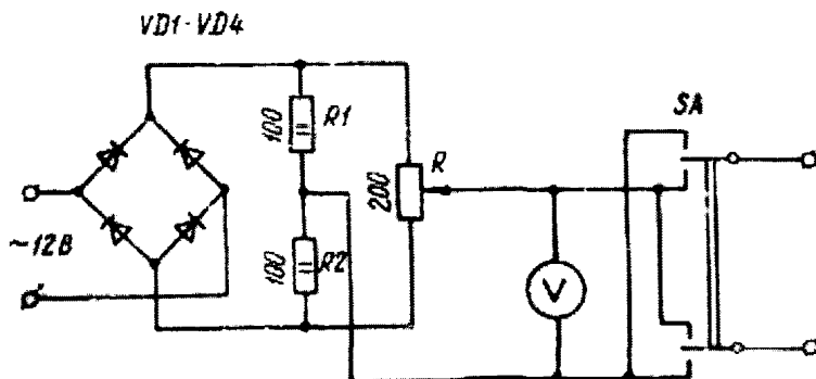
Рис. 16. Электрическая схема сигналов задания
