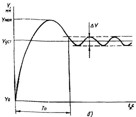
Рис. 14. Переходные процессы при холостом ходе агрегата: а - по частоте; б - по открытию НА
