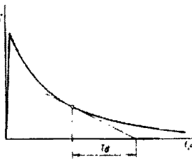
Рис.3. Переходная характеристика изодрома
