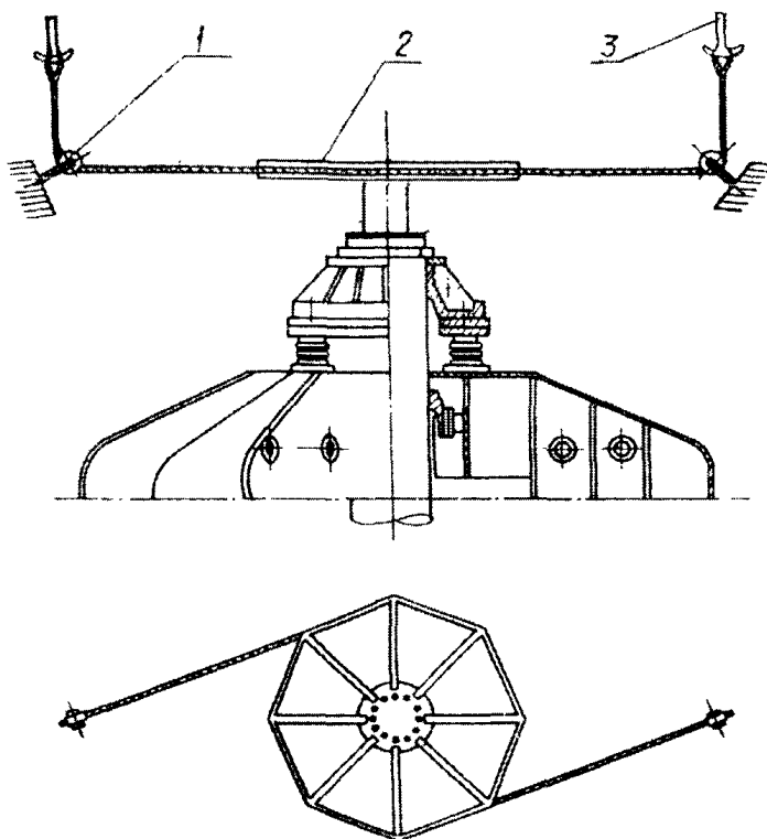
Рис.1. Схема поворота ротора агрегата: 1 - балка; 2 - приспособление для поворота ротора; 3 - гак мостового крана
