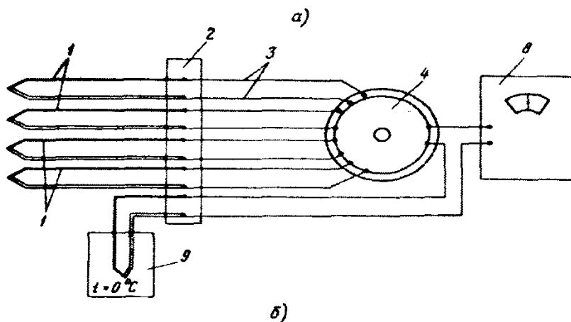
Рис.6. Схемы подключения термопар к потенциометрам: а - схема подключения термопар к электронному автоматическому потенциометру ЗПИ-09М; б - схема подключения термопар к переносному потенциометру III; 1 - рабочая термопара; 2 - панель зажимов; 3 - медные соединительные провода; 4 - переключатель; 5 - регистрирующий орган; 6 - усилитель; 7 - компенсационная термопара; 8 - потенциометр; 9 - термостат
