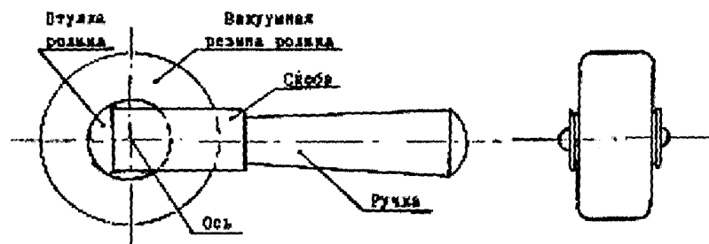
Рис. 3 РОЛИК ДЛЯ ПРИКАТЫВАНИЯ ТЕРМОЗИНТЕКОВ.
