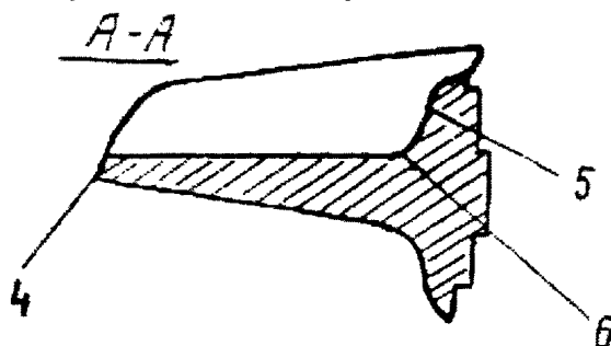
Рис.2. Схема лопасти рабочего колеса поворотно-лопастной гидротурбины с указанием основных мест контроля. 1 - входная кромка; 2 - монтажное отверстие; 3 - выходная кромка; 4 - периферийная кромка; 5 -
