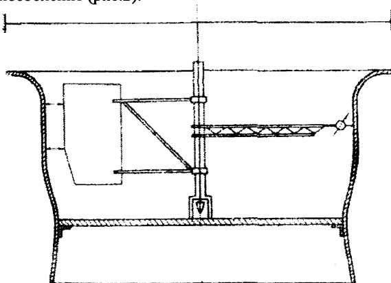
Рис.1. Проверка размеров камеры рабочего колеса с помощью струны
