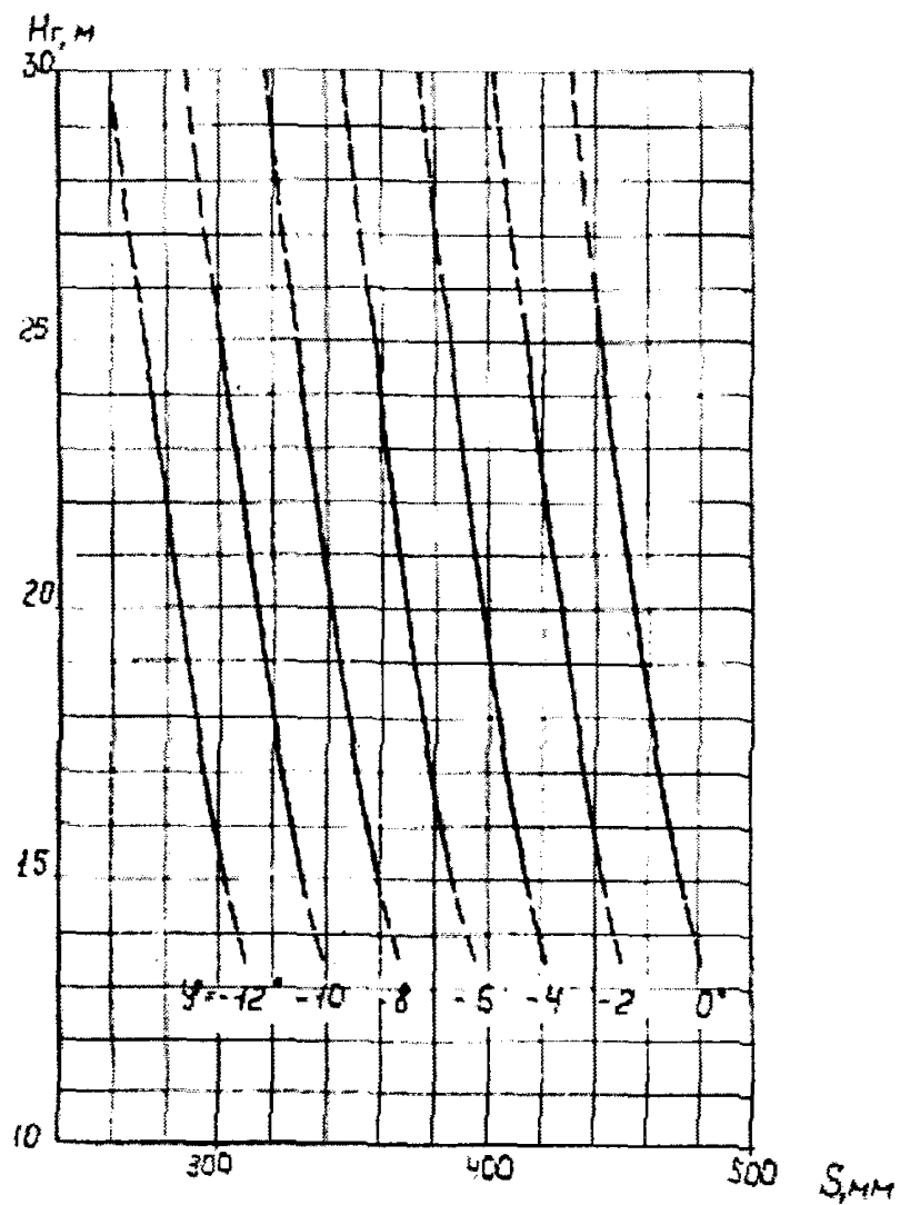
Рис.26. Графики линий равных углов в координатах H_g - S
