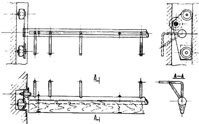
Рис. 9. Однорядная вертушечная рама
