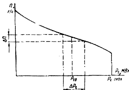
Рис.6. Статическая характеристика регулирования
