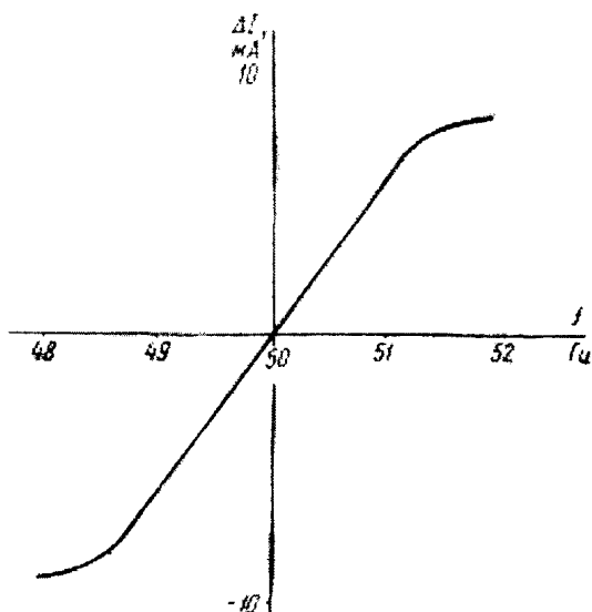
Рис. 8. Характеристика усилителя по входу частоты.
