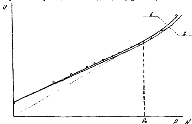
Рис.18. Расходная характеристика гидроагрегата (1) и турбины (2)
