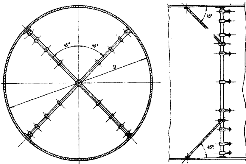
Рис.11. Стационарная рама
