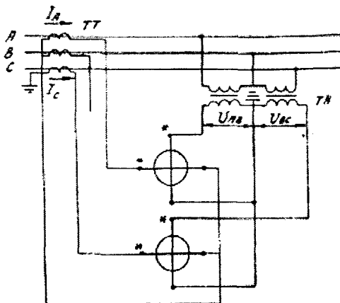
Рис.4. Схема измерения активной мощности в трехфазных цепях двумя однофазными ваттметрами
