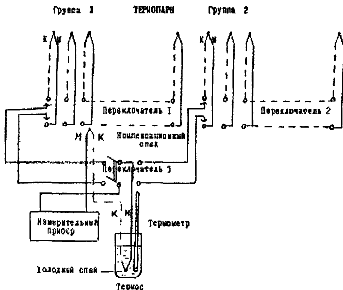
РИС.1 СХЕМА ИЗМЕРЕНИЯ ТЕМПЕРАТУРЫ ФАЗ ОБМОТКИ СТАТОРА ГИДРОГЕНЕРАТОРА ПРИ ПОМОЩИ ТЕРМОПАР
