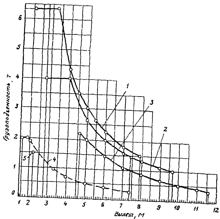
Рис. 11. Кривые грузоподъемности крана КС-2571А-1: на стрелах: 1 — на стреле 9 м; 2 — на стреле 10,8 м; 3 — на стреле 10,8 м с гуськом 2,2 м; 4 — на стреле 7,3 м; 5 — в статичном положении; 6 — при передвижении с грузом на крюке
