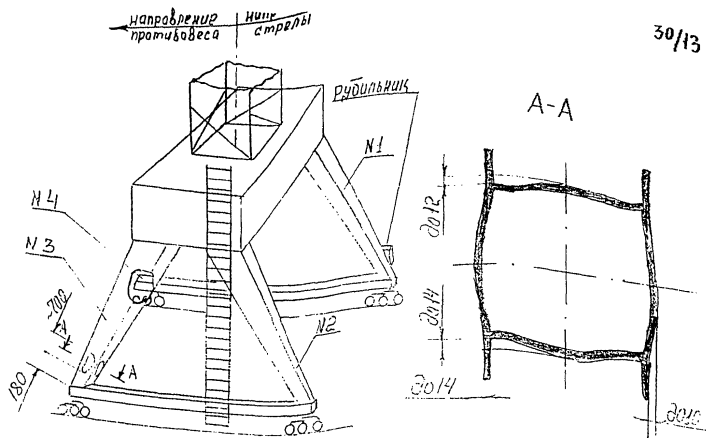
Рис. 1. Схема расположения дефектной стойки портала.
