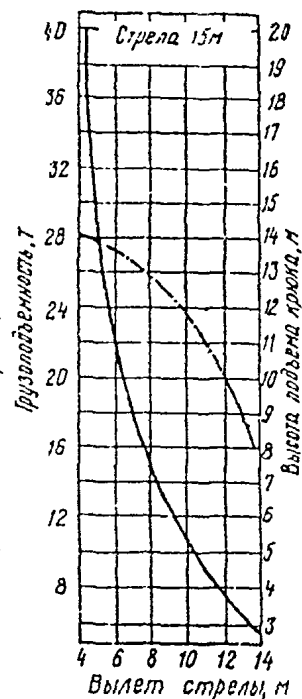
Грузовысотные характеристики крана КС-5363В с УПГ
