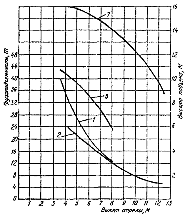
Грузовысотные характеристики крана КС-6471А:
