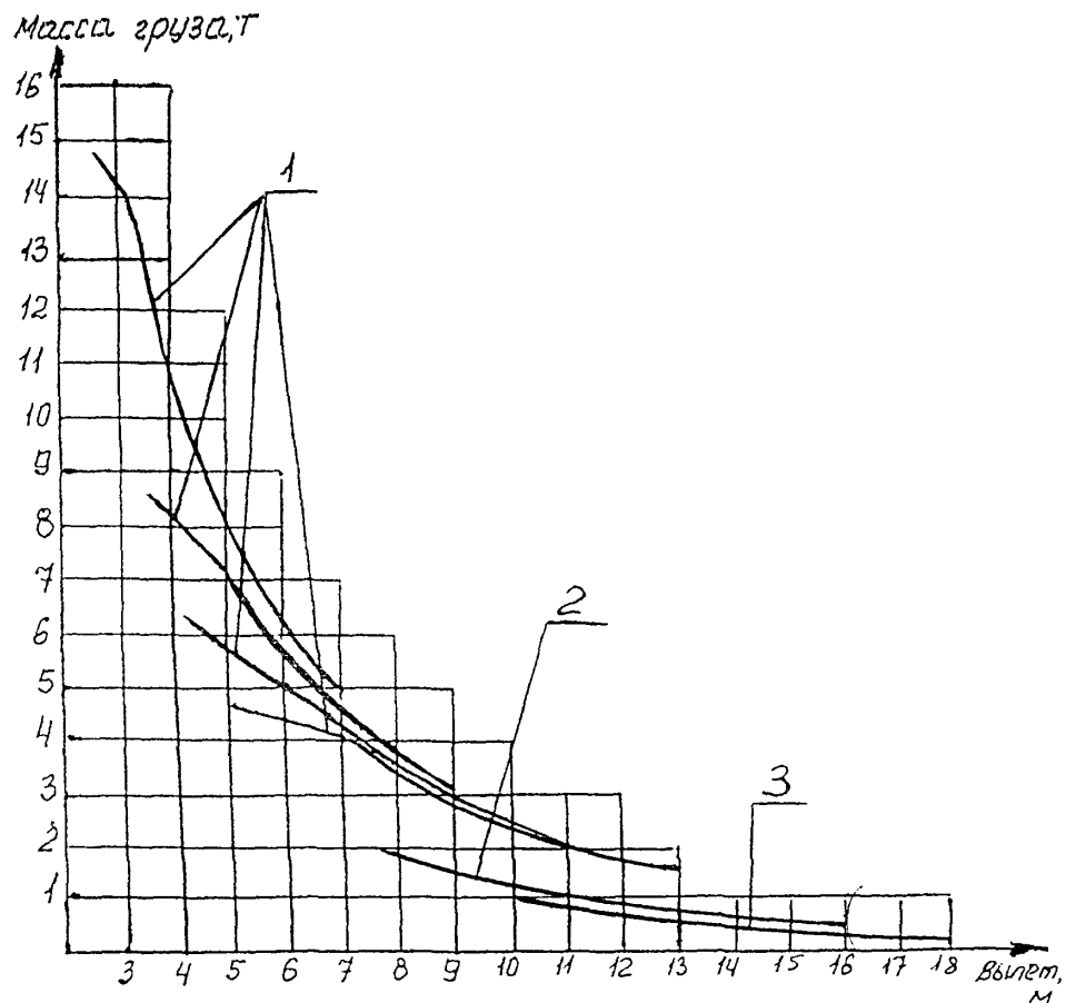
Рис. 7. Диаграмма грузовых характеристик крана КС-3577-4
