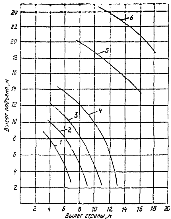
Кривые высоты подъема крюка крана КС-3577 (КС-3577-3-1). 1 — на стреле 8 м; 2 — на стреле 10 м; 3 — на стреле 12 м; 4 — на стреле 14 м; 5 — на стреле 14 м с гуськом 7 м; 6 на стреле 14 м с гуськом 7 м и вставкой 4,5 м
