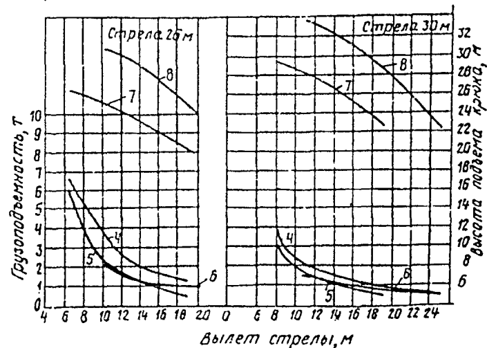
Грузовысотные характеристики крана КС-4562:
