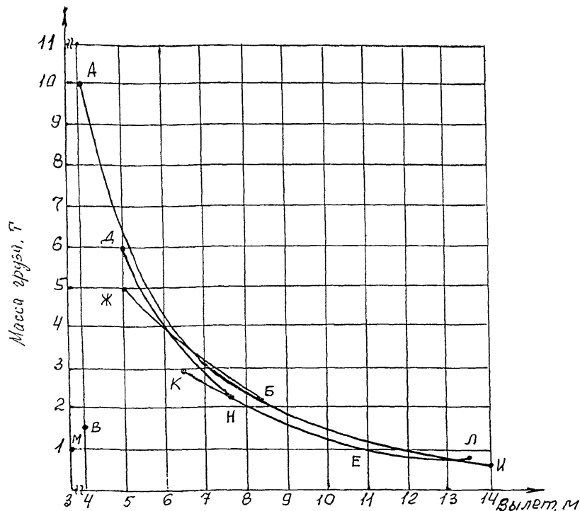
Рис. 5. Диаграмма грузовых характеристик стрелового крана СМК-101А
