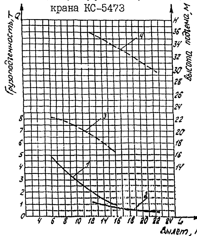
Грузовысотные характеристики (Диаграмма грузоподъемности и высоты подъема для стрелы с удлинителем 8 м ( \alpha = 0^\circ ) и неуправляемым гуськом 1 м ( \alpha = 31^\circ ))
