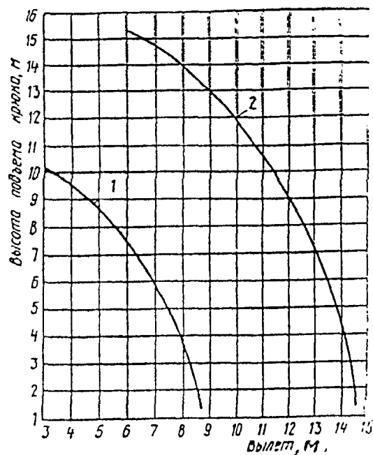
Высота подъема крюка крана КС-3575А 1 — на стреле 9,5 м; 2 — на стреле 15,5 м
