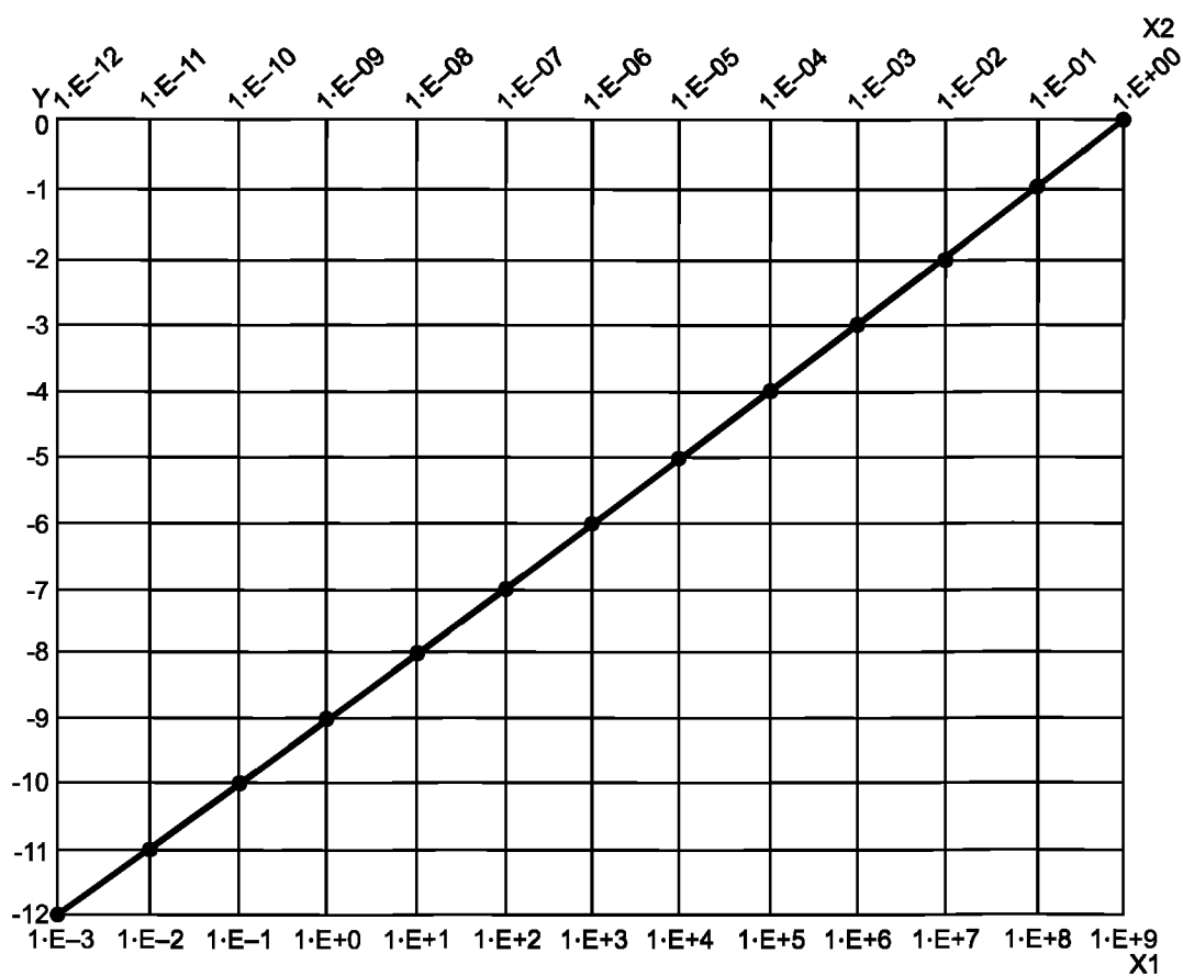
Рисунок 1 — Классы ИСО-АМС в зависимости от концентрации загрязнений
