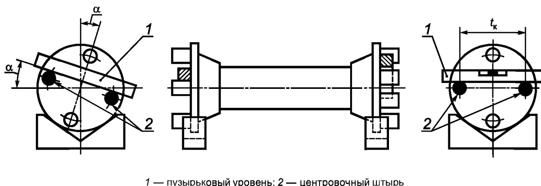
1 — пузырьковый уровень; 2 — центровочный штырь
