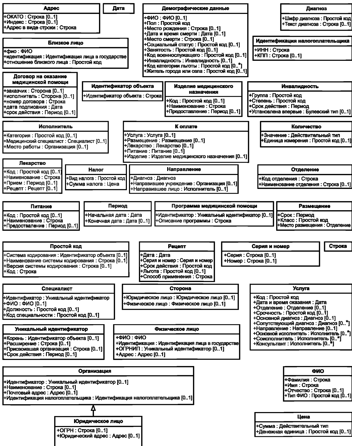
Рисунок А.2 — Вспомогательные классы
