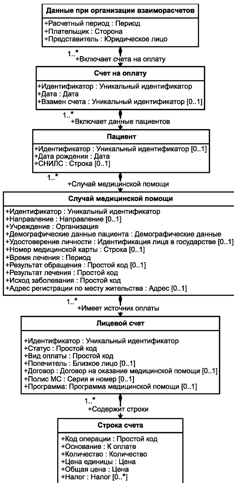
Рисунок А.1 — Данные при организации взаиморасчетов
