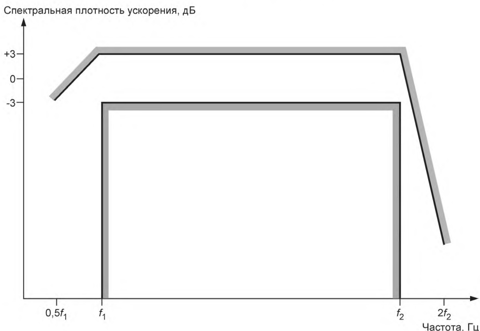
Рисунок 1 — Границы спектральной плотности ускорения (см. также 5.1.1)
