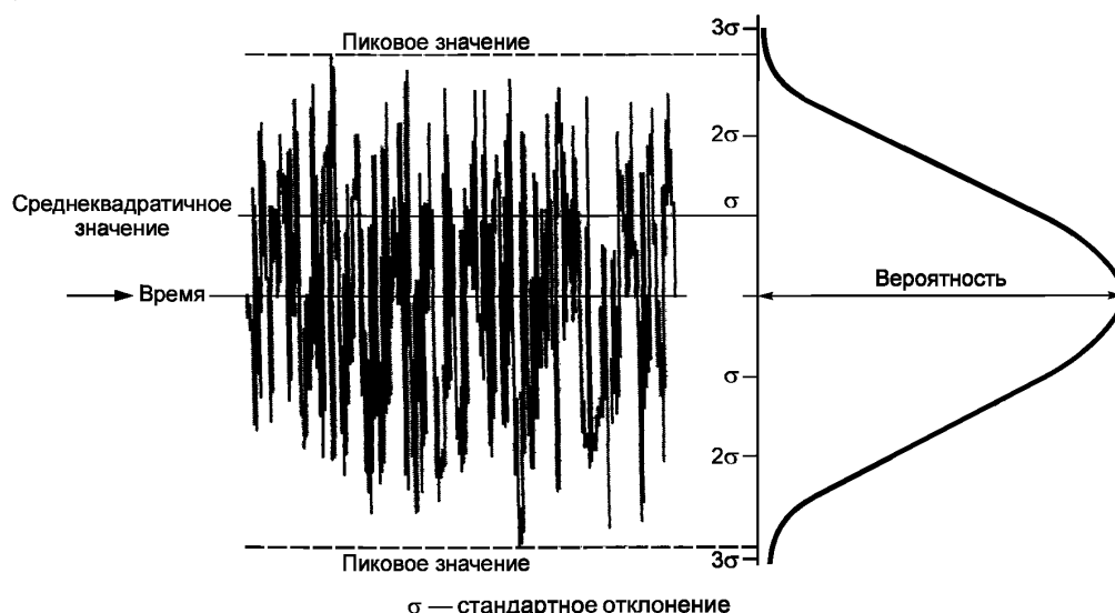
Рисунок 2 — Случайный сигнал, близкий к нормальному, с заданным уровнем отсеки
