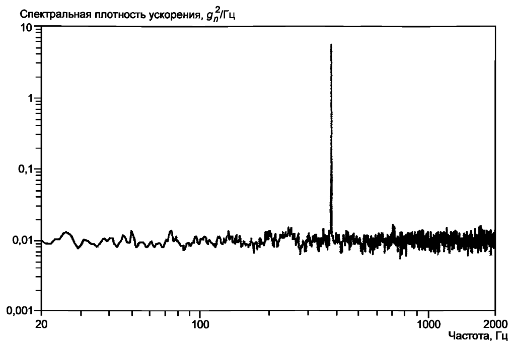
Рисунок А.2 — Гармонический сигнал на частоте 380 Гц
