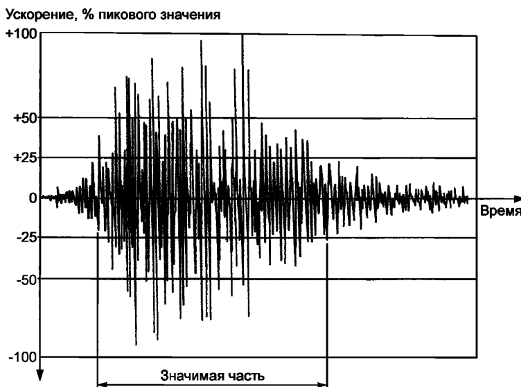
Рисунок 4 — Типичная форма временного сигнала возбуждения
