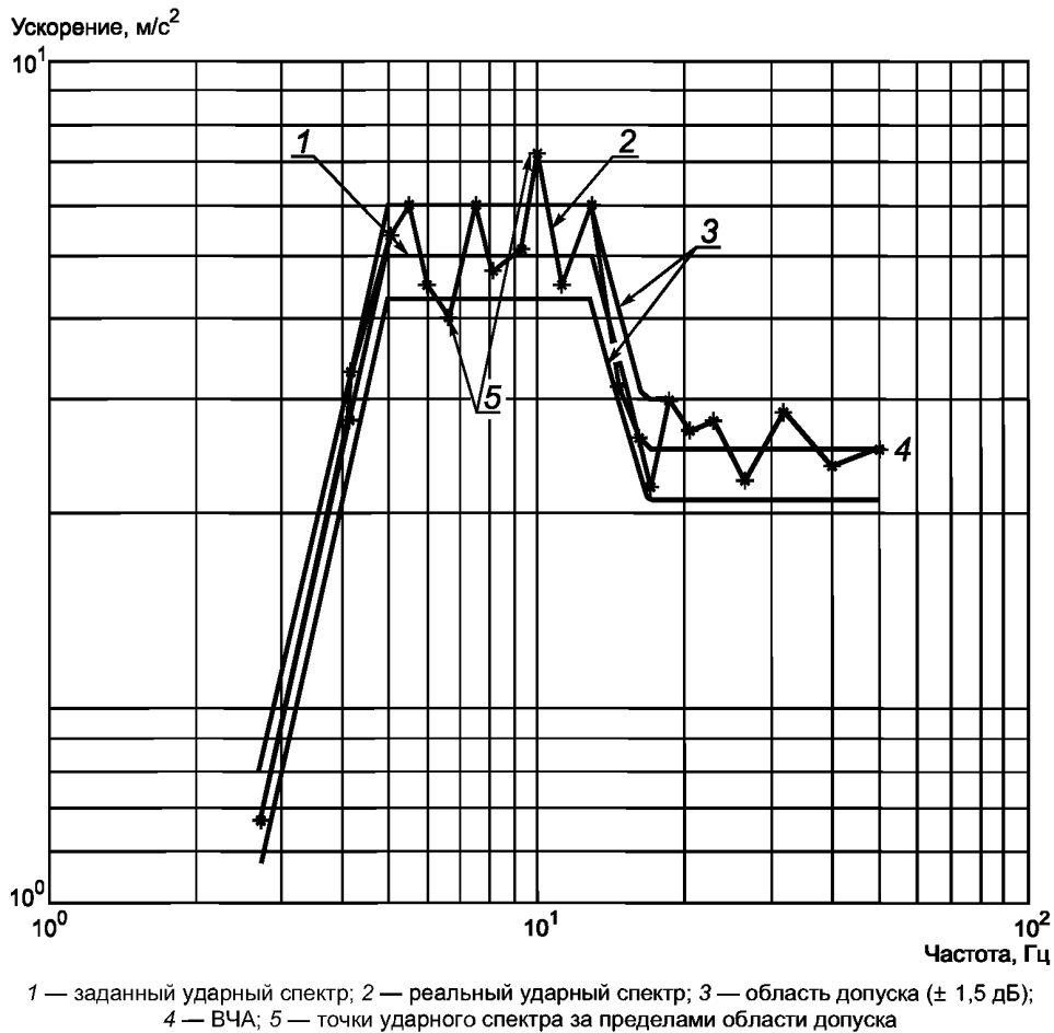
Рисунок 3 — Типичный график ударного спектра (в логарифмическом масштабе)
