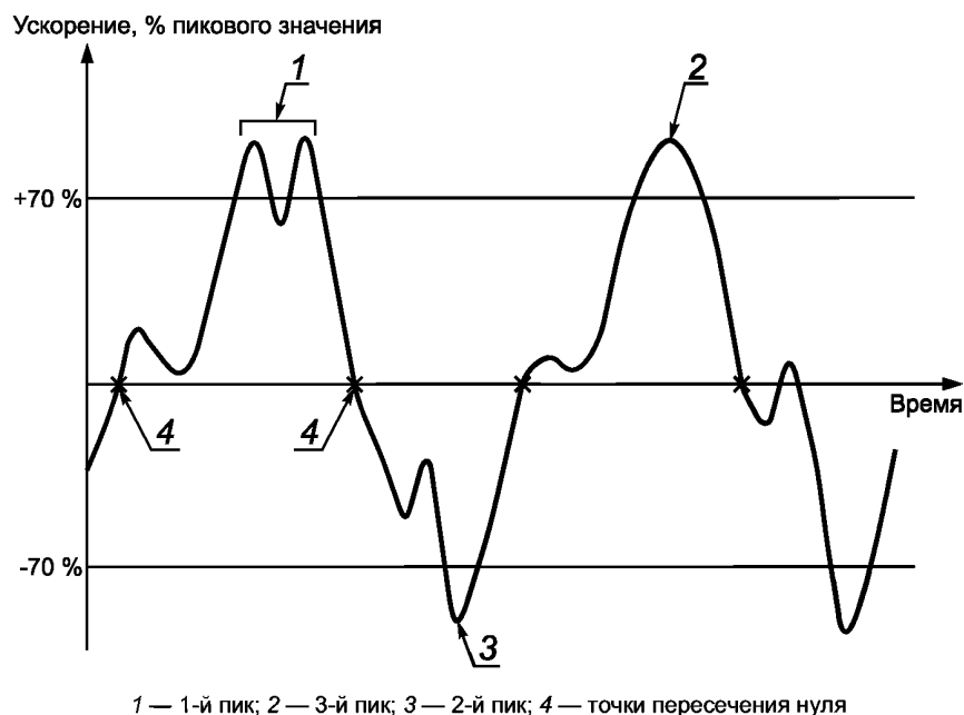
Рисунок 2 — Пример идентификации пиков отклика, превышающих пороговое значение (70 %)
