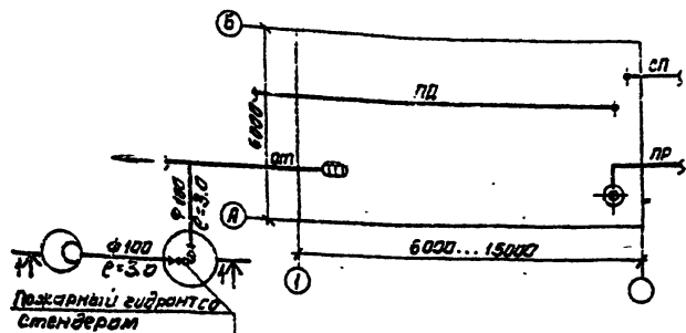
План резервуара емк. 100...300 м 3
