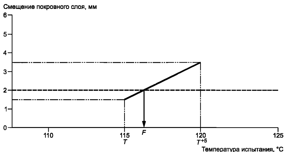
Рисунок 2 — Пример определения предельного значения теплостойкости интерполяцией
