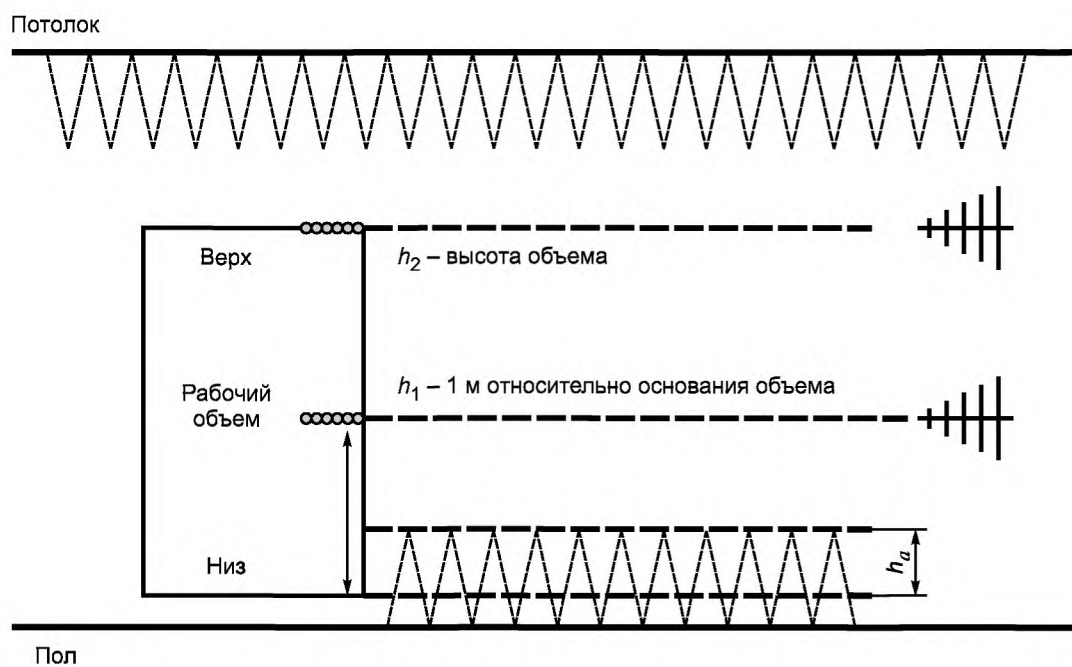
Рисунок 16 — Позиции при измерении КСВ н в горизонтальной плоскости (см. 8.2.2.2.1)
