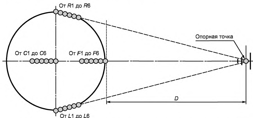
Рисунок 16 — Позиции при измерении КСВ н в горизонтальной плоскости (см. 8.2.2.2.1)
