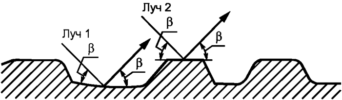
Рисунок 1 — Критерий шероховатости поверхности пластины заземления (по Релею)
