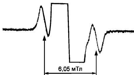
Рисунок А.2 — Спектр ЭПР фисташковой скорлупы, получившей дозу облучения 4,0 кГр; видна характерная пара линий радикала целлюлозы с расстоянием между ними (6,05 \pm 0,05) \text{ мТл}
