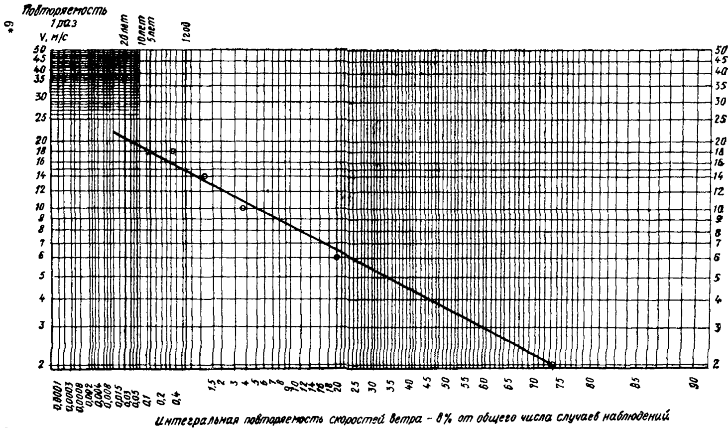
Рис. 5. Номограмма для определения скоростей ветра различной вероятности. Северное направление ветра (Москва, Сельскохозяйственная академия)
