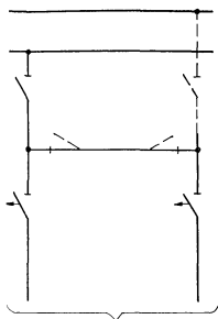
к трансформаторам а) схема 110, 220-4
