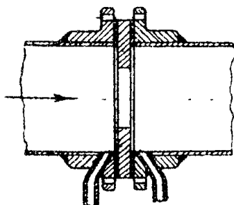
Бескамерная диафрагма
