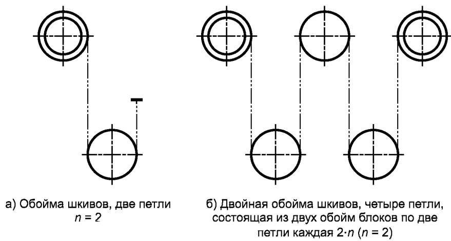
Рисунок D.3 — Обоймы блоков
