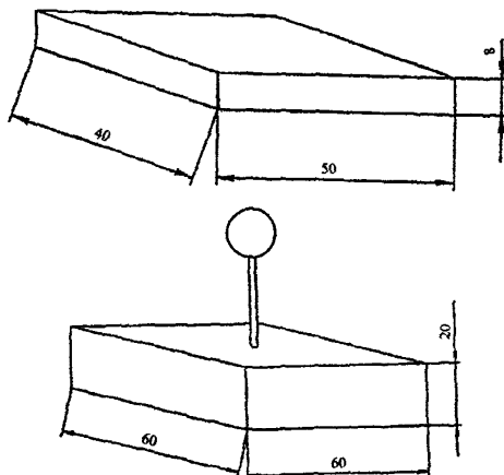
Рис. 2. Магнитный блок и крышка
