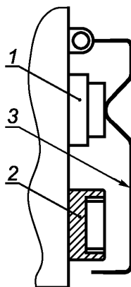
1 — кнопка «Выкл.»; 2 — кнопка «Вкл.»; 3 — защитный кожух
