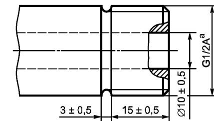
Рисунок 1 — Входной порт для клемм датчика температуры
