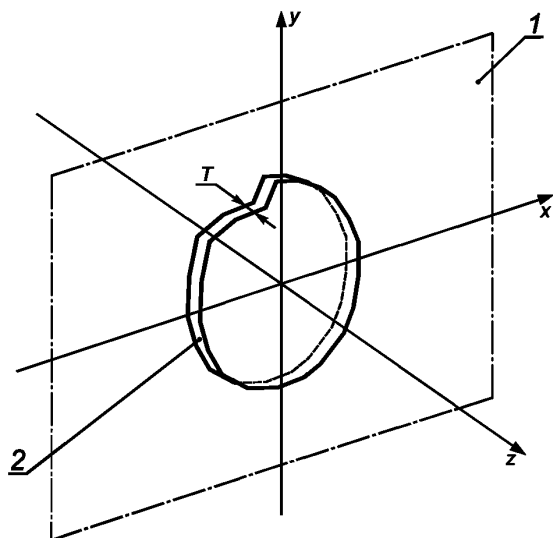
1 — томографическая плоскость; 2 — фантом
