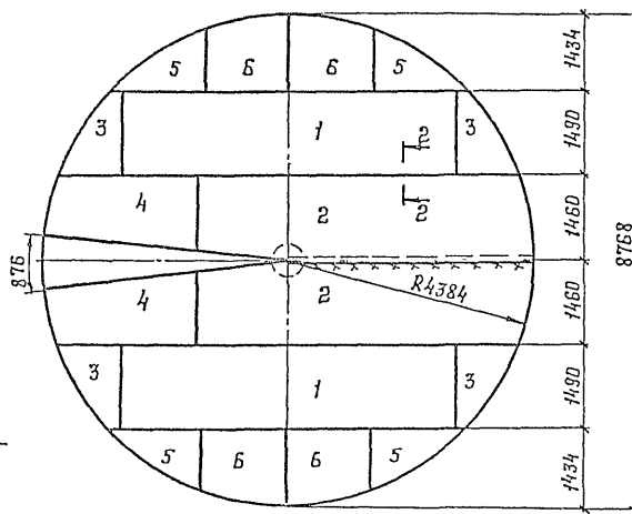
Развертка оболочки
