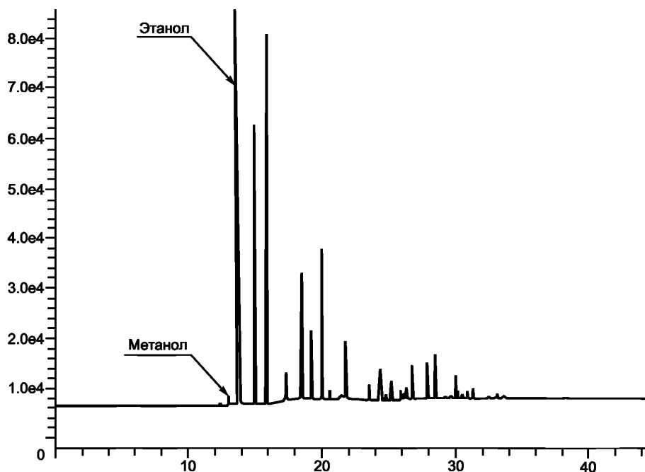
Рисунок 1 — Пример хроматограммы
