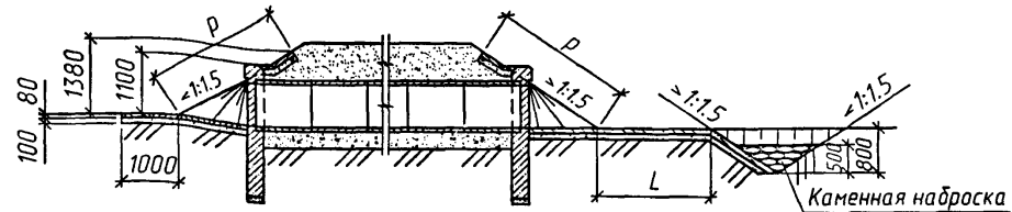
Укрепление блоками П-1 Входной оголовок Разрез по оси трубы Выходной оголовок
