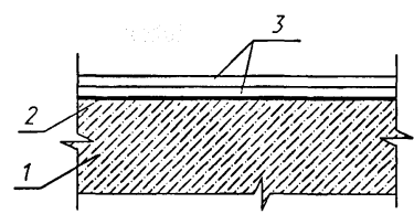
Гидроизоляция битумная мастичная неармированная
