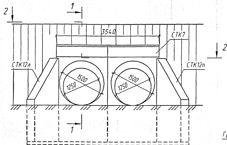
Фасад
