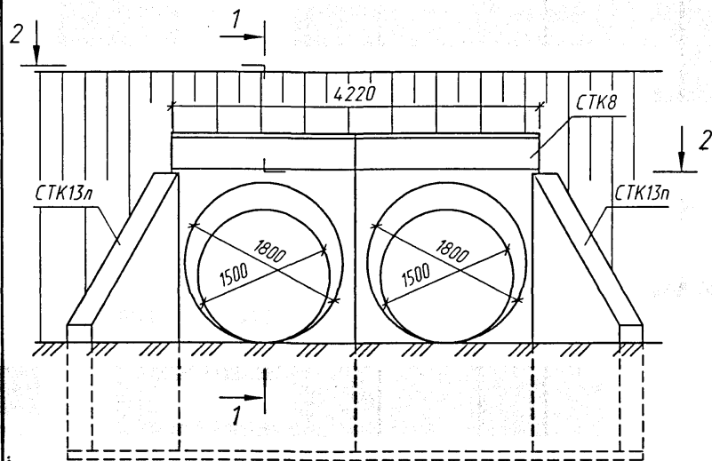
Фасад
