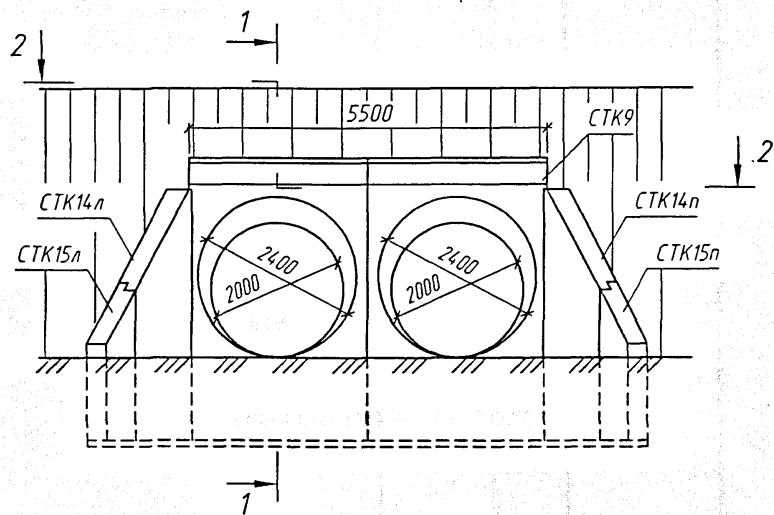
Фасад
