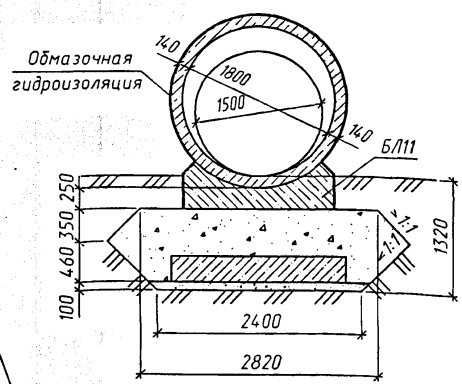
3-3 (насыпь не показана)
