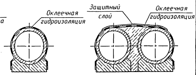
Устройство стыка конического звена с портовой стенкой (при оклеечной гидроизоляции)
