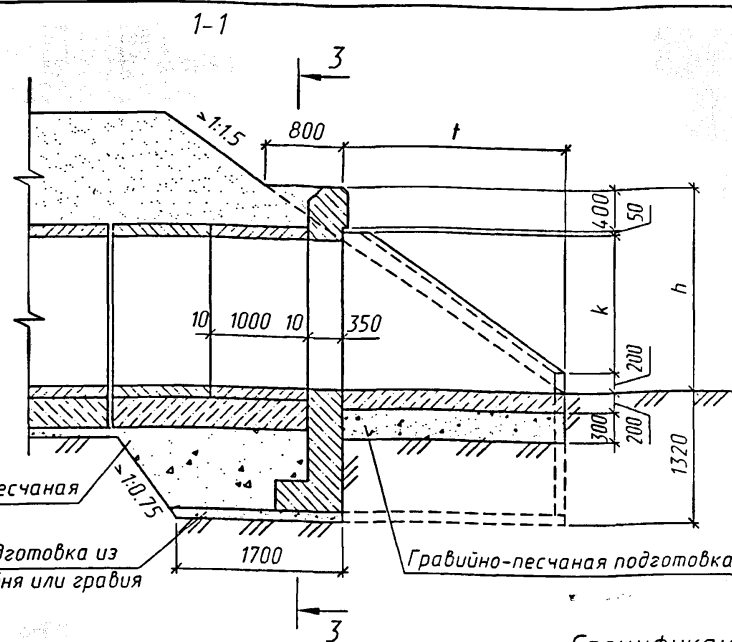
Размеры, мм
