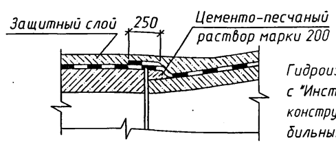
Сопряжение гидроизоляции стыка звеньев оголовка и тела трубы
