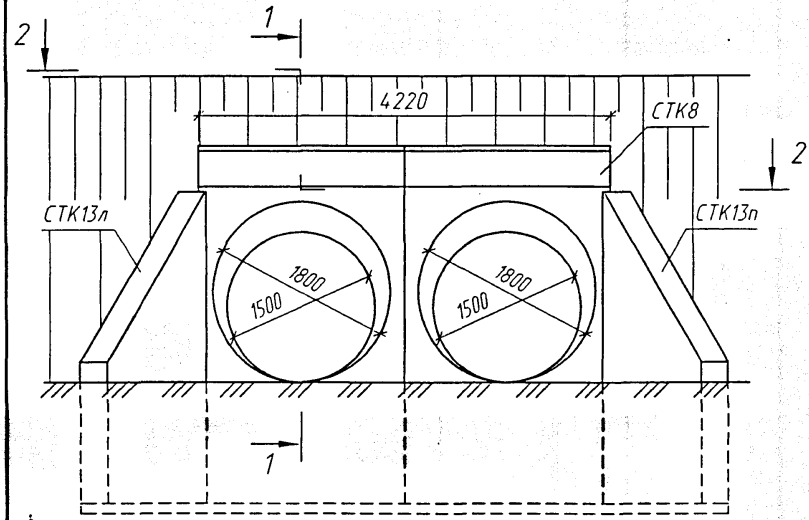
Фасад
