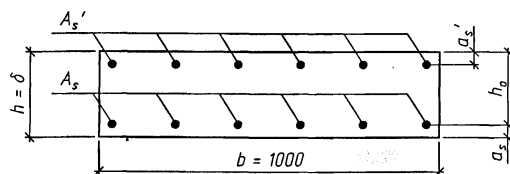
Расчетное сечение
