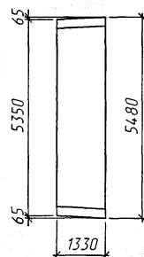
План фундамента (1:100)
