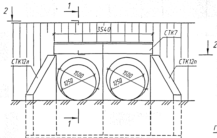
Фасад
