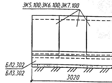
Секции труб
