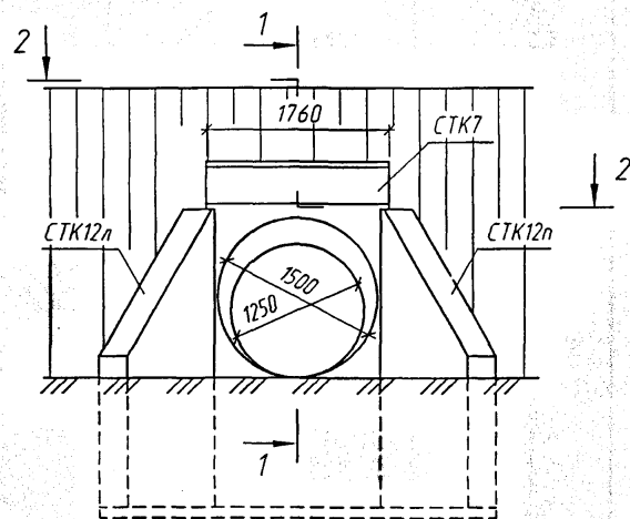
Фасад
