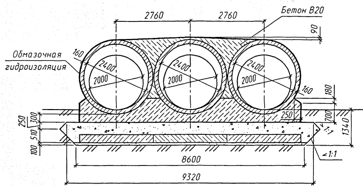
3-3 (насыпь не показана)
