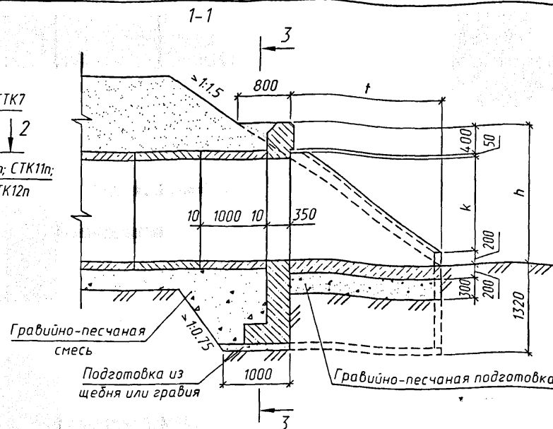
Размеры, мм
