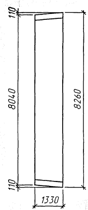
План фундамента (1:100)
