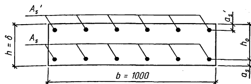
Расчетное сечение
