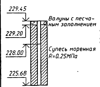
Скв. №12 ПК8+25 право от оси пути 8.0м
