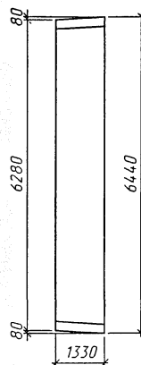
План фундамента (1:100)
