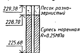
Скв.№31 ПК110+45 право от оси пути 8.0м
