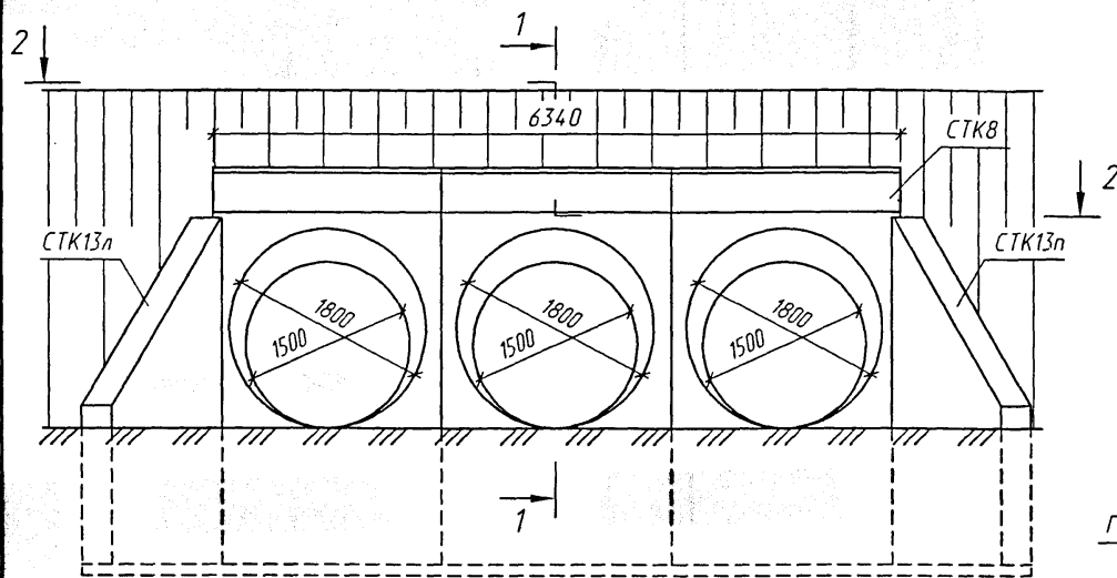
Фасад
