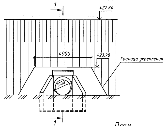
Фасад входного оголовка
