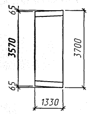
План фундамента (1:100)
