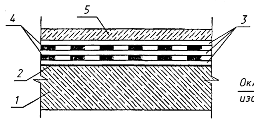
Гидроизоляция битумная мастичная неармированная
