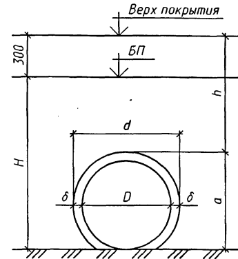
Расчетная схема
