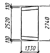
План фундамента (1:100)
