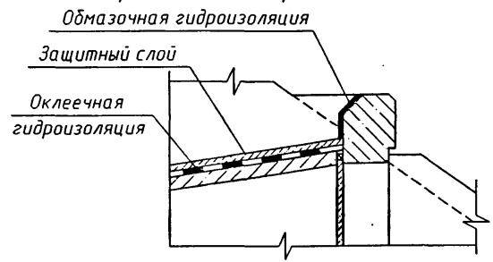
Устройство стыка конического звена с портовой стенкой (при обмазочной гидроизоляции)
