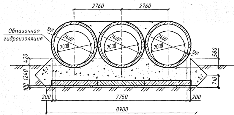
3-3 (насыпь не показана)
