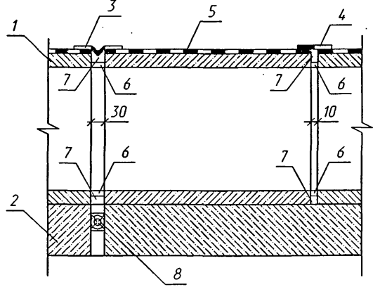
Гидроизоляция стыков звеньев и секций трубы
