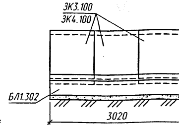
Секции труб
