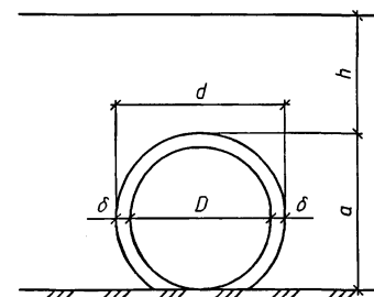
Расчетная схема
