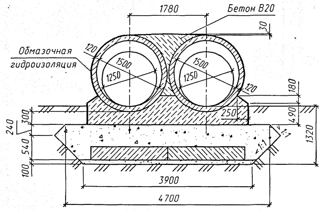
3-3 (насыпь не показана)
