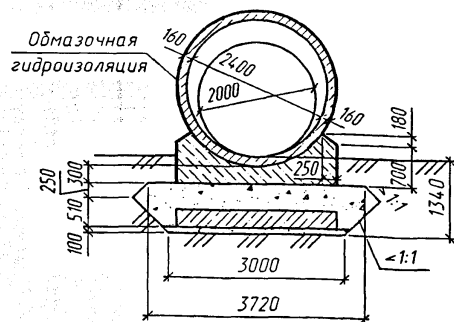
3-3 (насыпь не показана)
