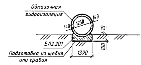
2-2 (насыпь не показана)
