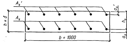
Расчетное сечение
