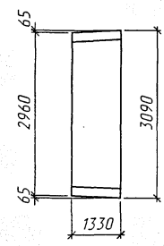
План фундамента (1:100)
