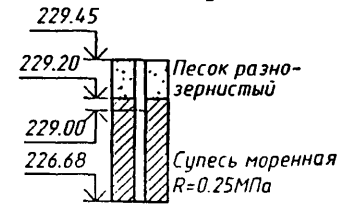
Скв.№30 ПК110+45 лево от оси пути 7.5м
