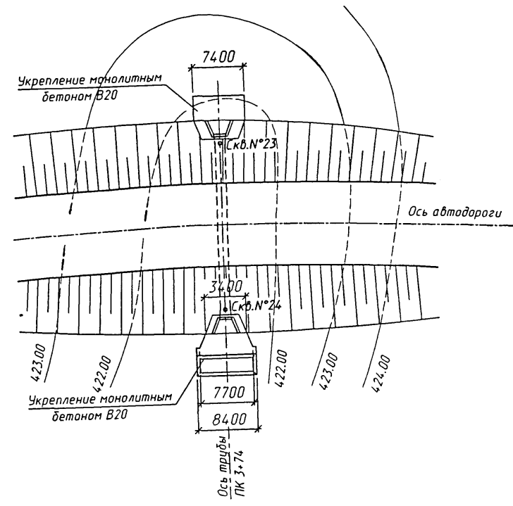
План (1:500)
