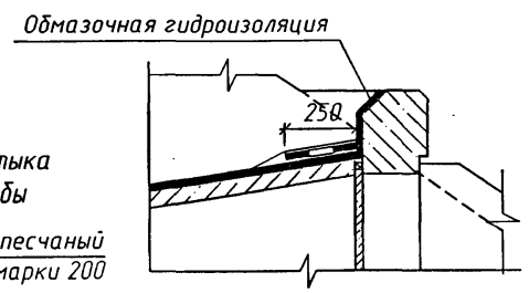
Устройство стыка конического звена с портовой стенкой (при обмазочной гидроизоляции)
