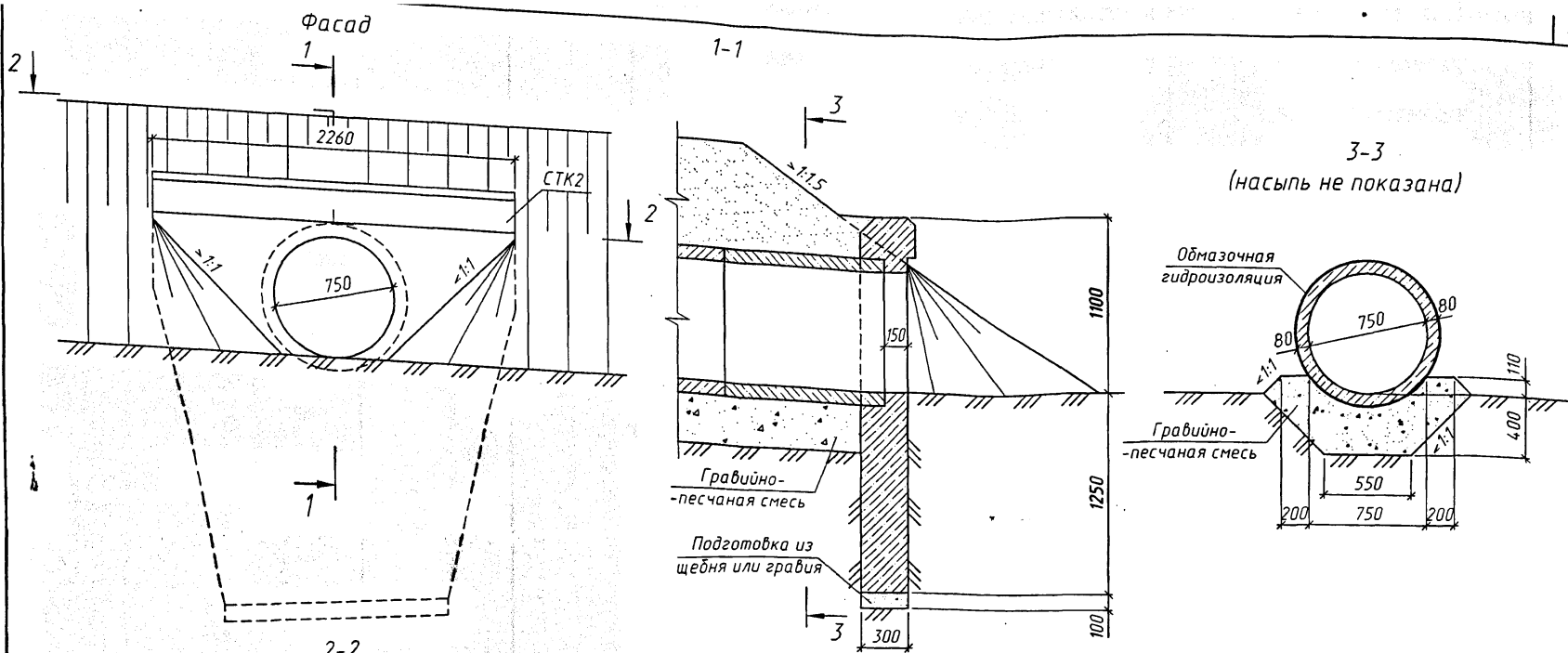
Спецификация блоков на оголовок
