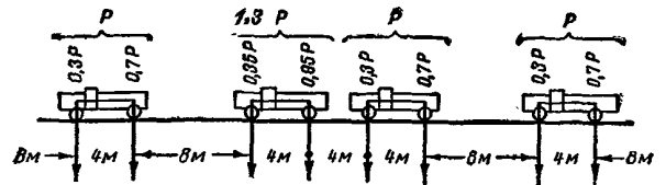
Рис. 2. Нормативная автомобильная нагрузка по схемам Н-13, Н-10 и Н-8 ( P принимается равным 13, 10 и 8 т)
