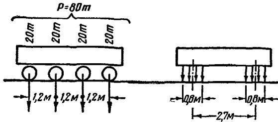
Рис. 3. Нормативная колесная нагрузка по схеме НК-80
