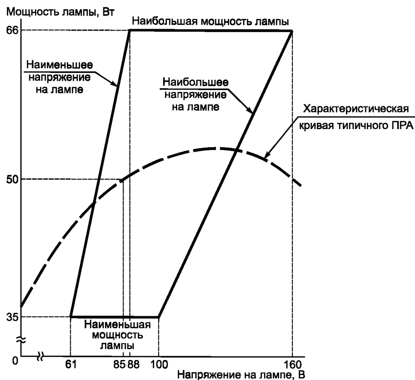
Рисунок Н.9 — Предельные рабочие характеристики лампы номинальной мощностью 50 Вт с трубчатой прозрачной, эллипсоидной прозрачной или с диффузным покрытием колбой
