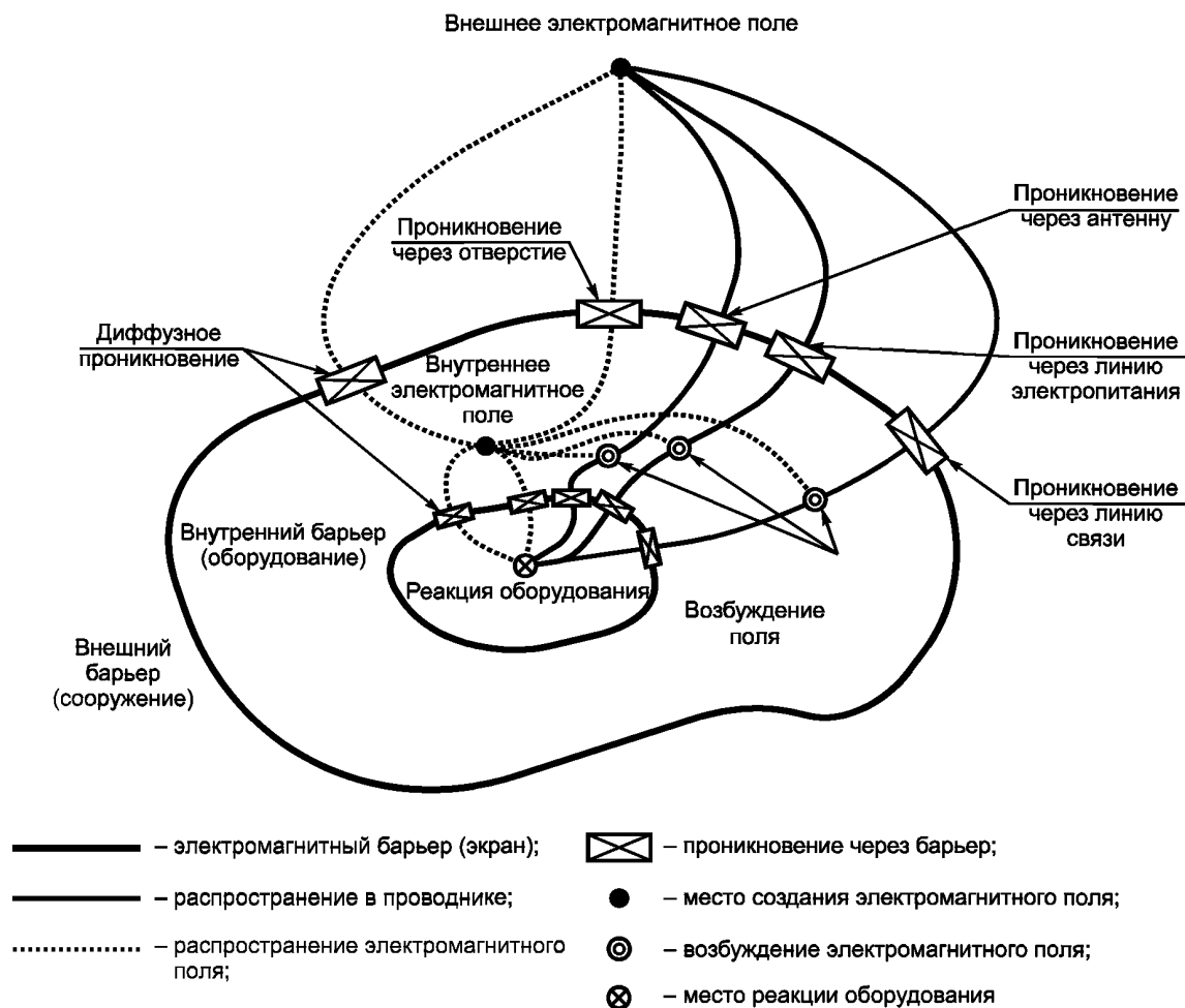
Рисунок 6 — Топологическая схема простой системы, представленной на рисунке 5
