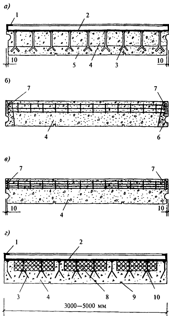
а — двухслойная панель на металлическом листе; б — панель с окаймляющим каркасом из тяжелого жаростойкого бетона; в — панель с окаймляющим арматурным каркасом; г — панель со стальными анкерами и эффективной теплоизоляцией; 1 — уголок жесткости панели; 2 — металлический лист; 3 — анкер; 4 — легкий жаростойкий бетон с D1100 и менее; 5 — легкий жаростойкий бетон с D1200 и более; 6 — окаймляющий каркас из тяжелого жаростойкого бетона; 7 — арматурный каркас; 8 — эффективная теплоизоляция; 9 — усадочный шов; 10 — шайба
