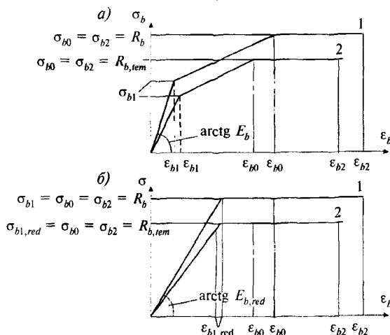
а — трехлинейная; б — двухлинейная; 1 — при 20 °C; 2 — при нагреве
