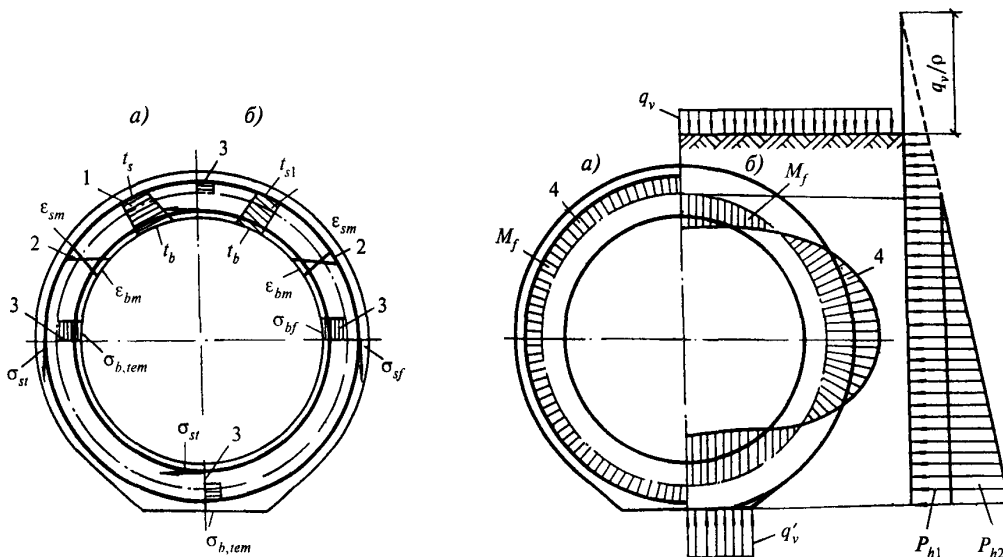
а — от воздействия температуры; б — от воздействия нагрузки; 1 — температур; 2 — деформаций; 3 — напряжений; 4 — усилий в подземном круглом железобетонном борове
