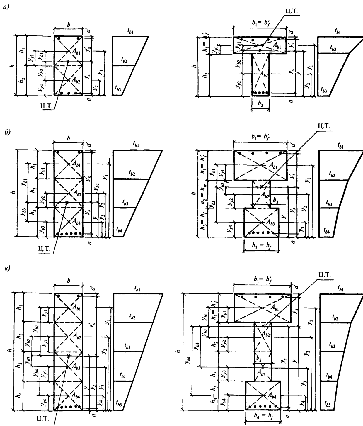
Рисунок 6.1 — Схемы разбивки на части по высоте прямоугольного, таврового и двутаврового сечения элементов
