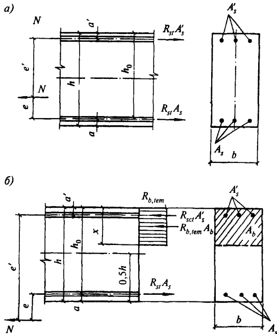
a — продольная сила N приложена между равнодействующими усилий в арматуре S и S' ; б — то же, за пределами расстояния между равнодействующими усилий в арматуре S и S'
