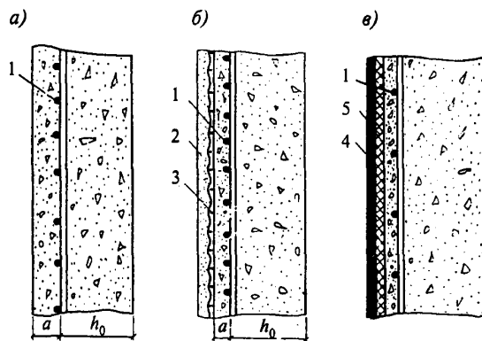
a — однослойная из сборного или монолитного железобетона; b — то же, с теплоизоляционной штукатуркой; в — то же, с теплоизоляцией и стальным кожухом; 1 — арматура; 2 — теплоизоляционная штукатурка; 3 — металлическая сетка; 4 — стальной кожух; 5 — теплоизоляция
