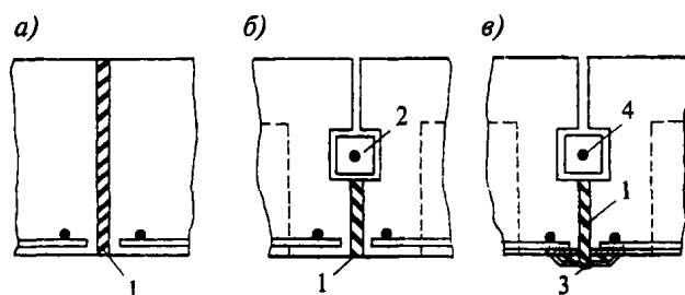
Рисунок 9.1 — Стыки элементов сборных конструкций из жаростойкого бетона
