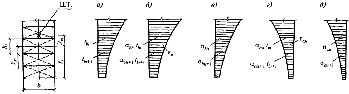
a — температуры бетона; b — деформации удлинения от нагрева; в — напряжения в бетоне от нагрева; г — деформации укорочения от остывания; д — напряжения в бетоне от остывания при нелинейном изменении температур по высоте бетонного сечения элементов. Ц.Т. — центр тяжести приведенного сечения
