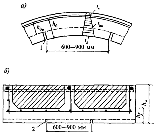
a — компенсационные; б — усадочные; 1 — компенсационный шов шириной 2—5 мм; 2 — усадочный шов глубиной 0,1h_f и шириной 2—3 мм
