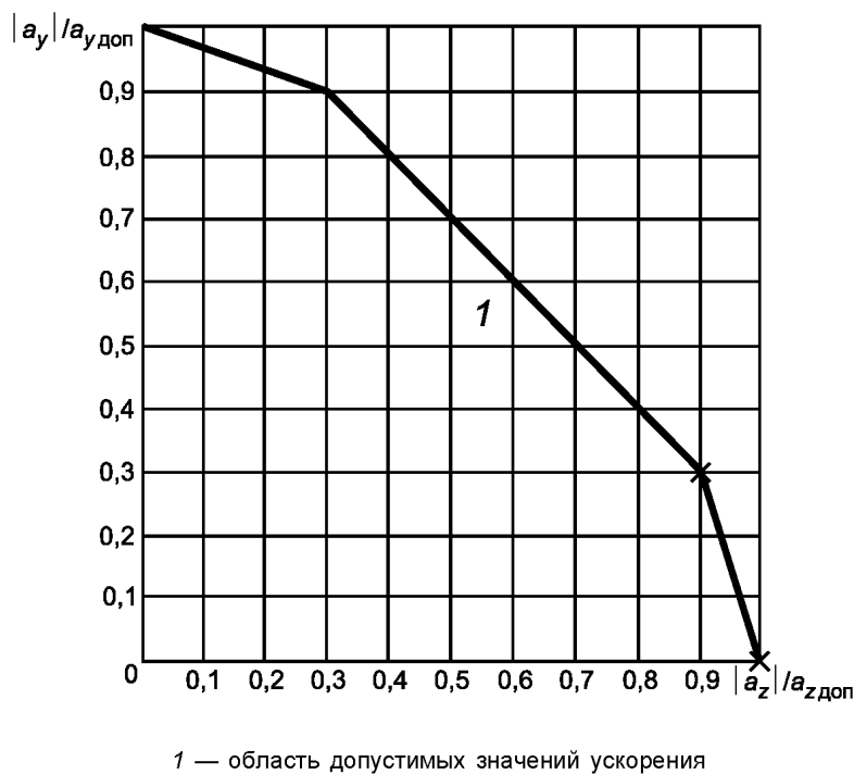
Рисунок Б.3 — Совместное воздействие ускорений |a_y| и |a_z|
