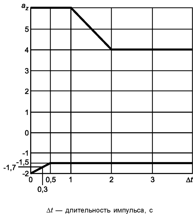
Рисунок Б.2 — Допустимое ускорение a_z в зависимости от длительности импульса
