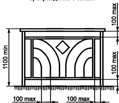
б) Ограждение с декоративными элементами
