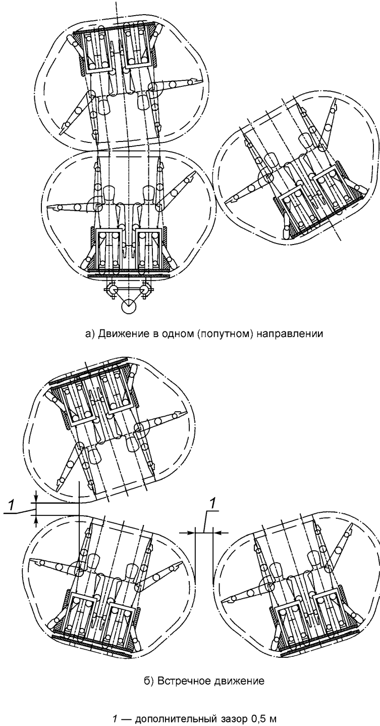
Рисунок 8 — Контуры безопасности для движущихся пассажирских модулей
