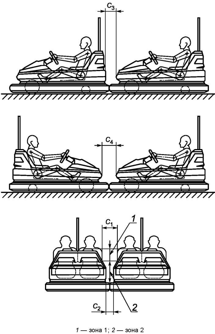
Рисунок 15 — Сталкивающиеся автомобили, лист 1
