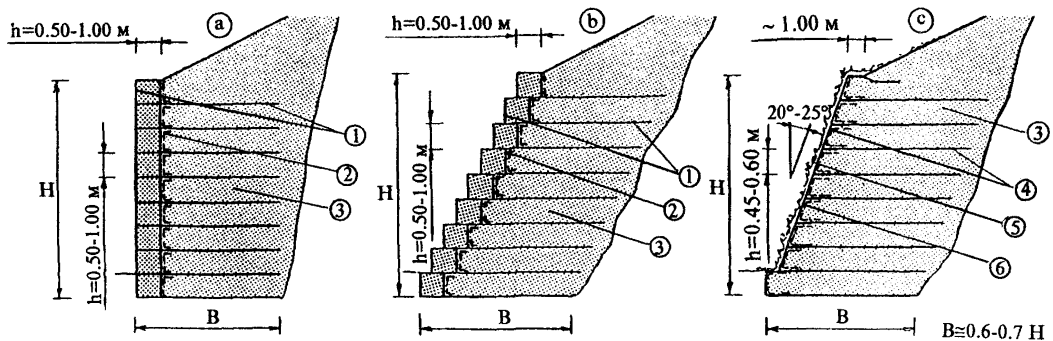
1 - Элемент системы Террамеш. 2 - Геотекстиль. 3 - Грунт засыпки. 4 - Элемент Зеленого Террамеша. 5 - Гидропосев. 6 - Биополотно.
