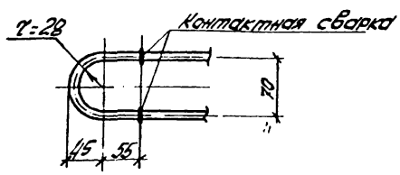
Деталь приварки поз. 71 к поз. 80
