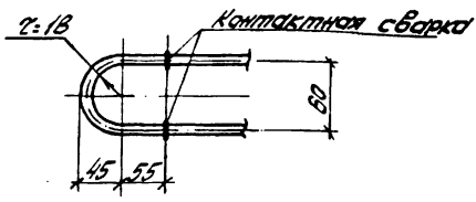
Деталь приварки поз. 84 к поз. 125
