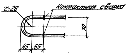
Деталь приварки поз. 71 к поз. 70
