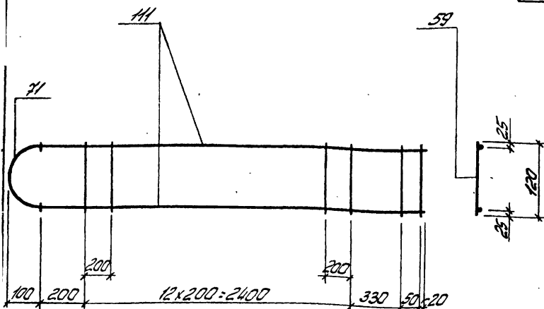
Деталь приварки поз. 71 к поз. III
