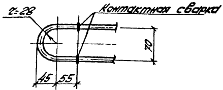
Деталь приварки поз. 71 к поз. 72
