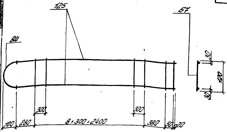
Деталь приварки поз. 84 к поз. 125
