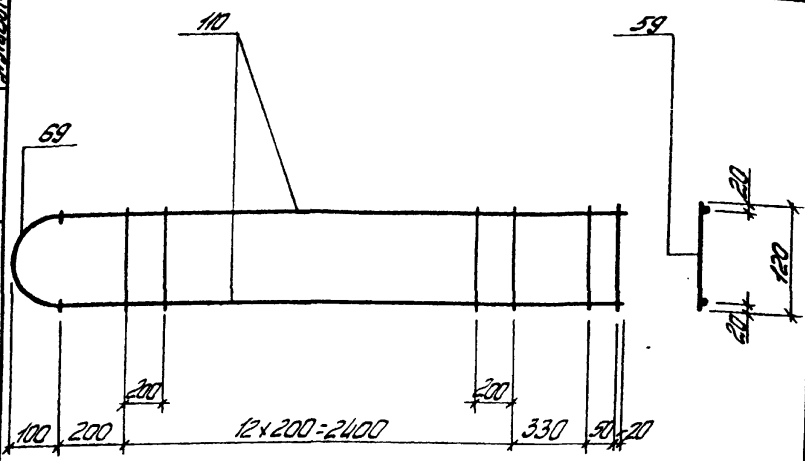
Деталь приварки поз. 69 к поз. 110
