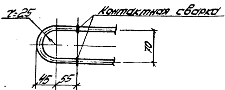
Деталь приварки поз. 78 к поз. 77
