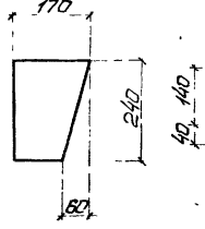
Деталь 10 а/BC139
