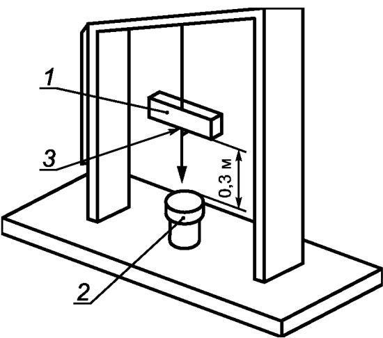
1 — стальная плита; 2 — образец; 3 — стальной пруток диаметром приблизительно 38 мм
