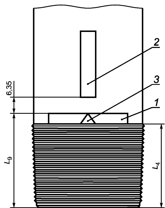
1 — полоса краской зеленого цвета; 2 — полоса краской на ниппельном конце шириной приблизительно 25 мм и длиной приблизительно 0,6 м, если муфта будет установлена изготовителем длиной не менее 100 мм; 3 — треугольное клеймо; L 4 — общая длина резьбы от торца трубы до конца сбега резьбы; L 9 — максимальная длина свинчивания: от торца трубы до вершины треугольного клейма
