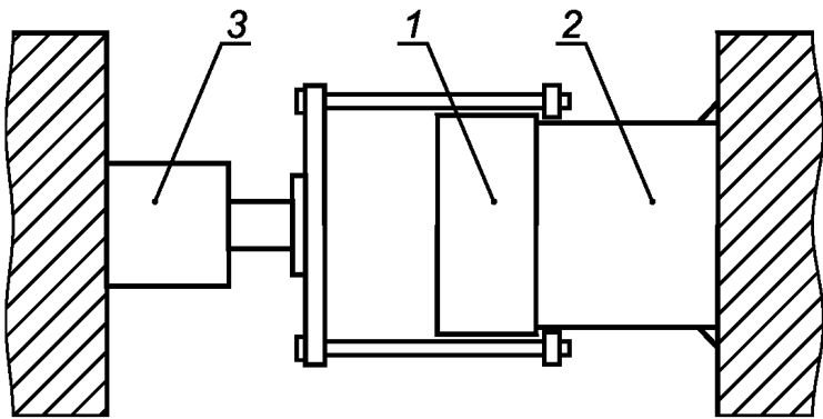
1 — резьбовая предохранительная деталь; 2 — участок трубы; 3 — гидроцилиндр
