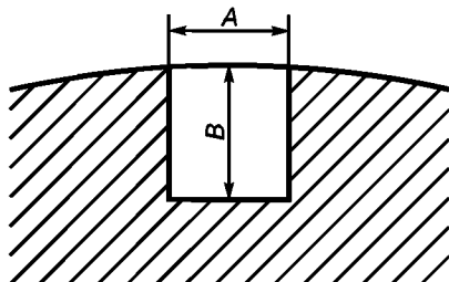
b – Надрез на наружной поверхности
