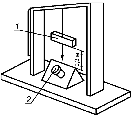
1 — стальная плита; 2 — образец
