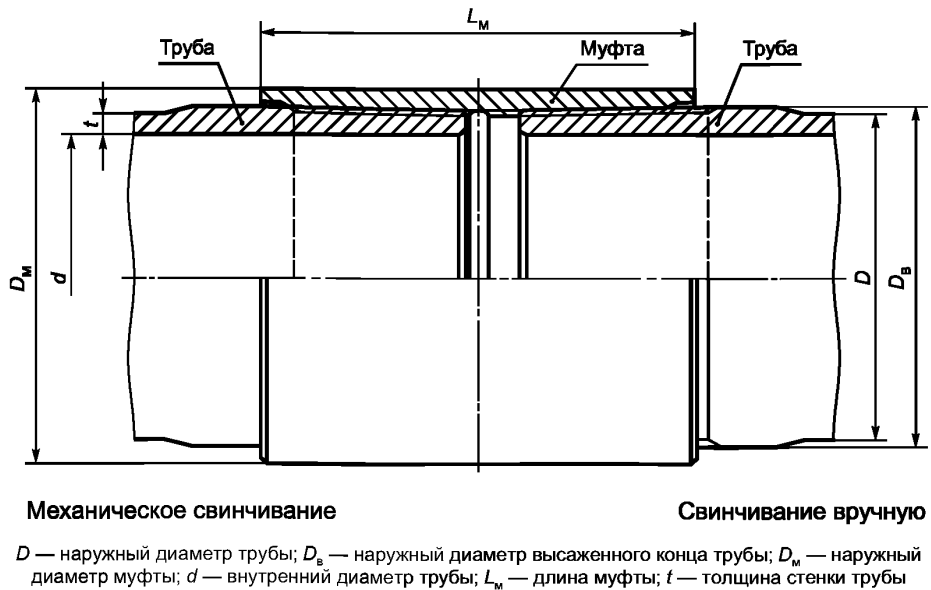
Рисунок 14 — Общий вид резьбового соединения НКТВ
