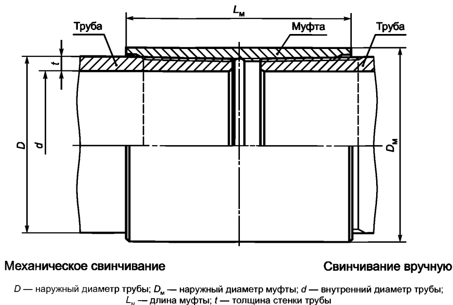
Рисунок 13 — Общий вид резьбового соединения НКТ
