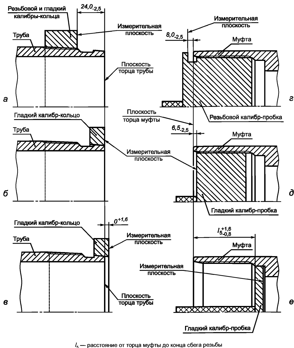
Рисунок 23 — Схема контроля калибрами резьбового соединения ОТТГ
