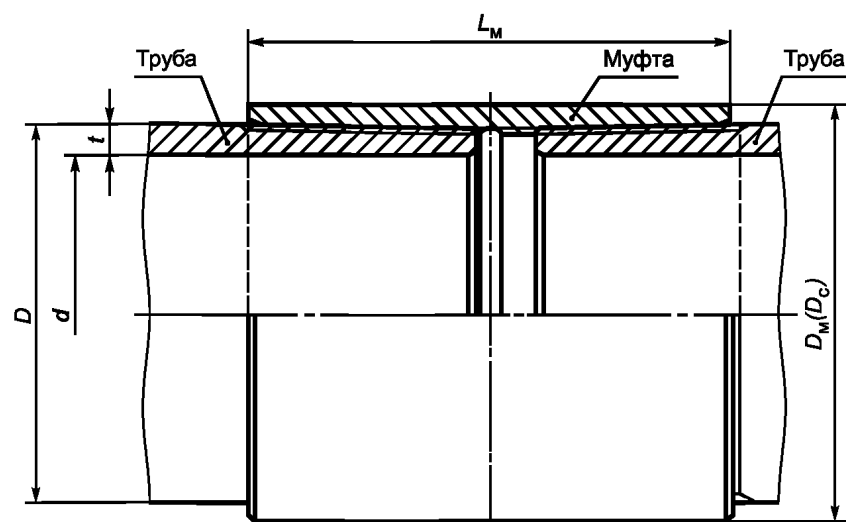
Механическое свинчивание
