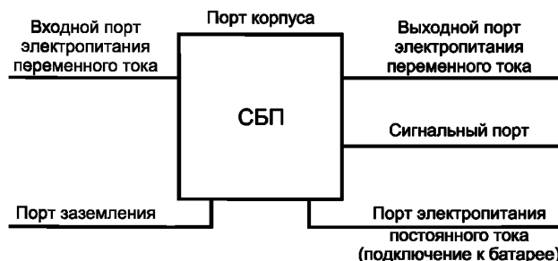
Рисунок 1 — Примеры портов СБП
