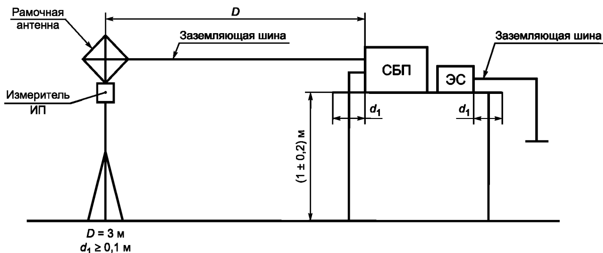
Рисунок В.1 — Схема испытаний СБП (настольное оборудование, измерение напряженности магнитного поля)
