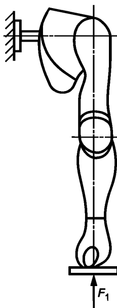
Рисунок 3 — Схема испытания на осевое нагружение концевой устройства
