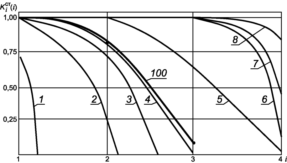
Рисунок А.2 — Кривая зависимости K_f(i) , нанесенная на серию тарировочных кривых
