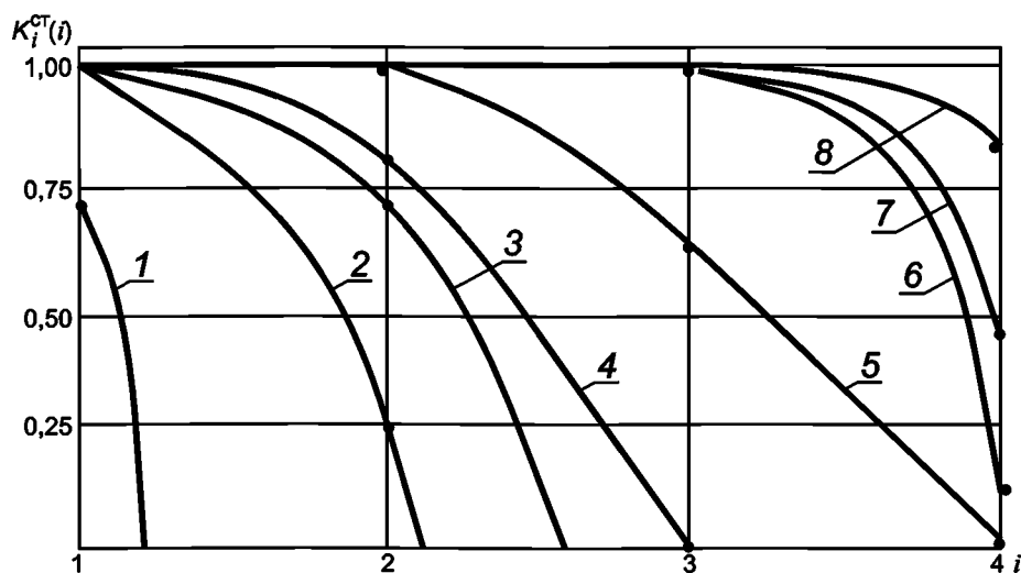
Рисунок А.1 — Серия тарировочных кривых K_i^{\text{СТ}}(i)
