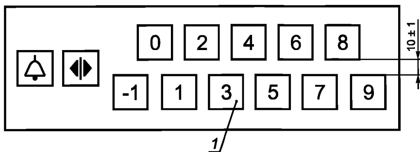
Рисунок В.3 — Пост управления в кабине при двухрядном горизонтальном расположении кнопок приказов
