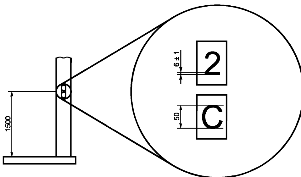
Рисунок А.2 — Размеры символов
