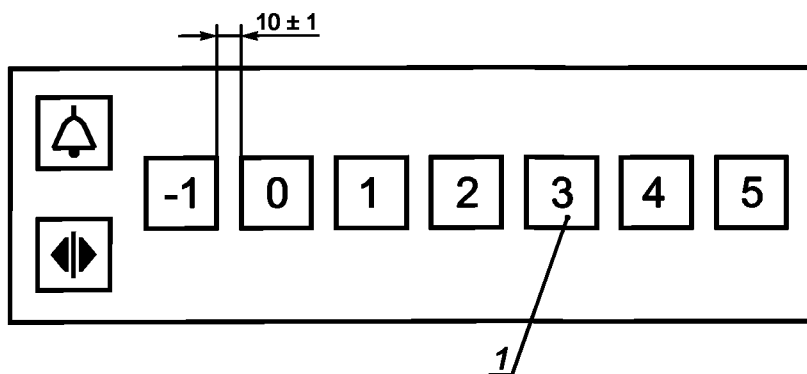
Рисунок В.2 — Пост управления в кабине при однорядном горизонтальном расположении кнопок приказов
