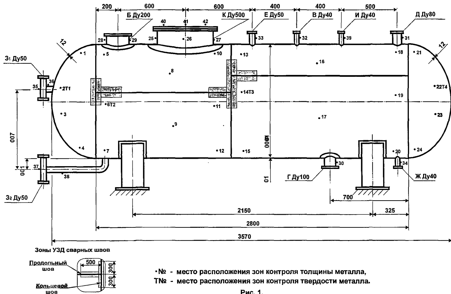
Схема распределения зон контроля корпуса емкости тех. поз. Е-6/1, зав. №9, рег. №НС-2925 М 1:15
