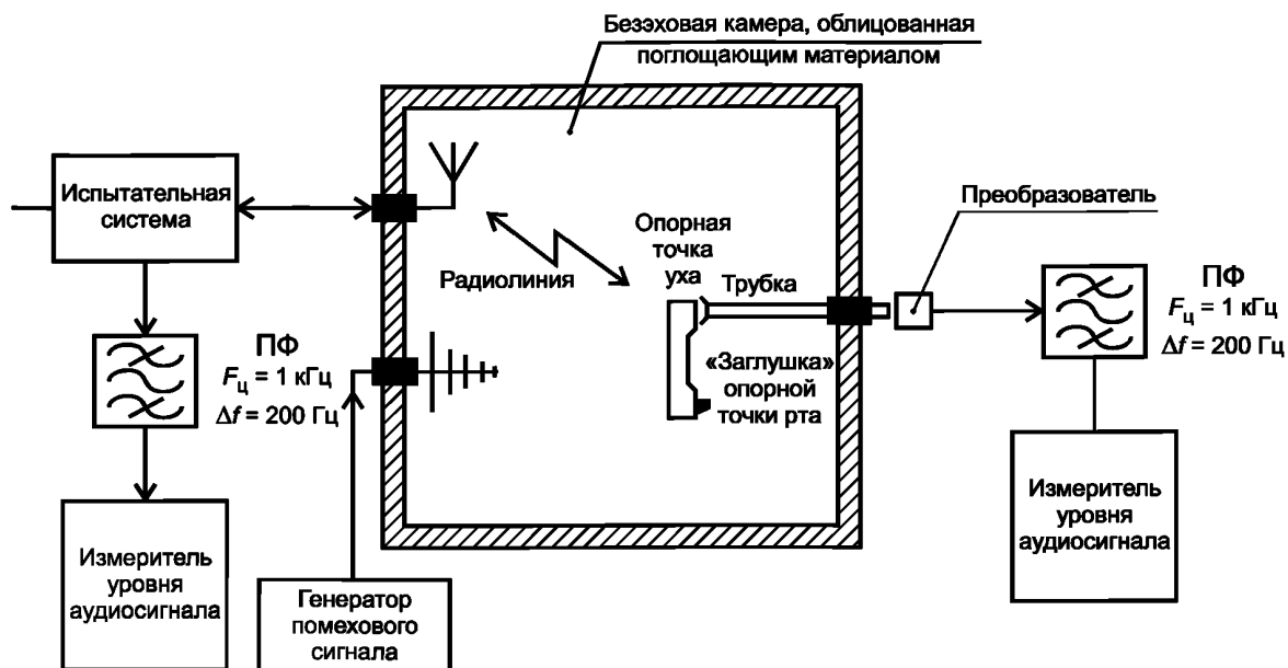
Рисунок 2 — Схема прохождения сигнала при испытаниях радиооборудования
