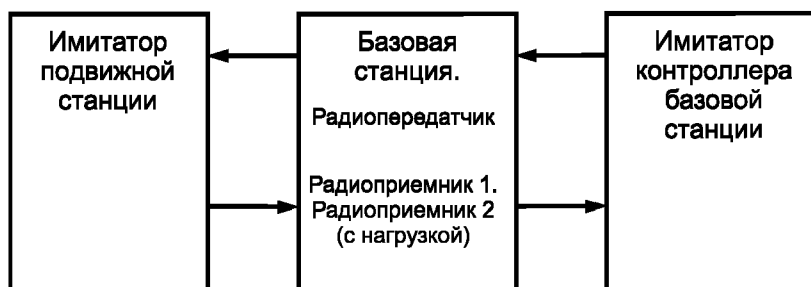
Рисунок 1 — Установление линии связи при испытаниях базовой станции на помехоустойчивость
