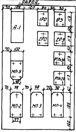
Задняя стенка шкафа при снятой
