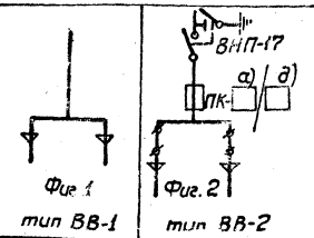
Схемы шкафов высоковольтных вводов
