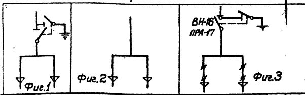
Схемы шкафов высоковольтных вводов
