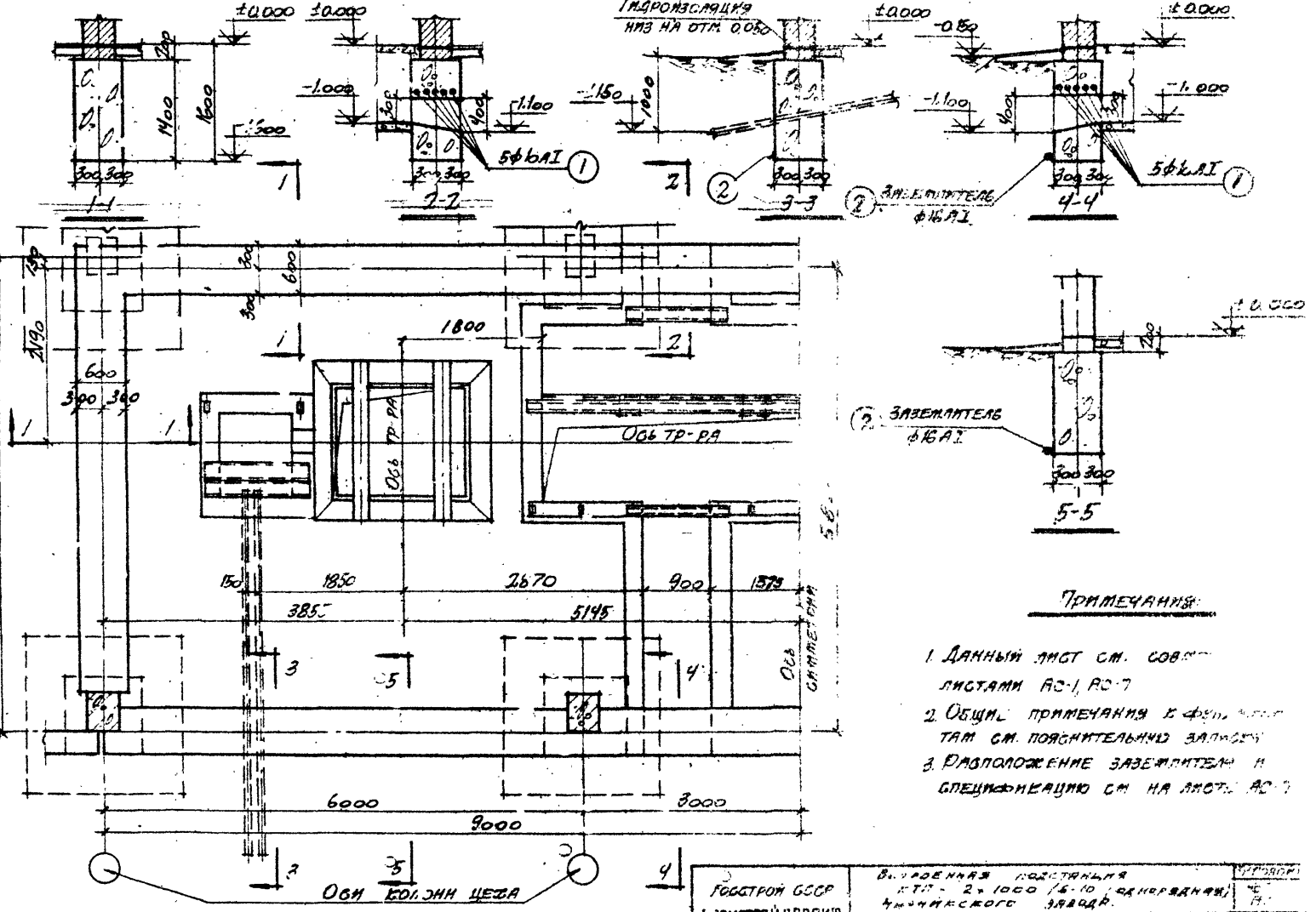
ПЛАН ФУНДАМЕНТОВ
