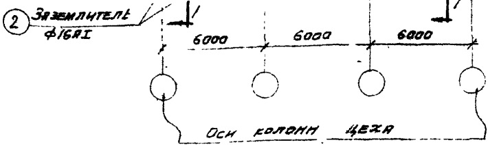
ПЛАН РАСПОЛОЖЕНИЯ ЗАЗЕМЛЯЮЩИХ ПРОВОДНИКОВ
