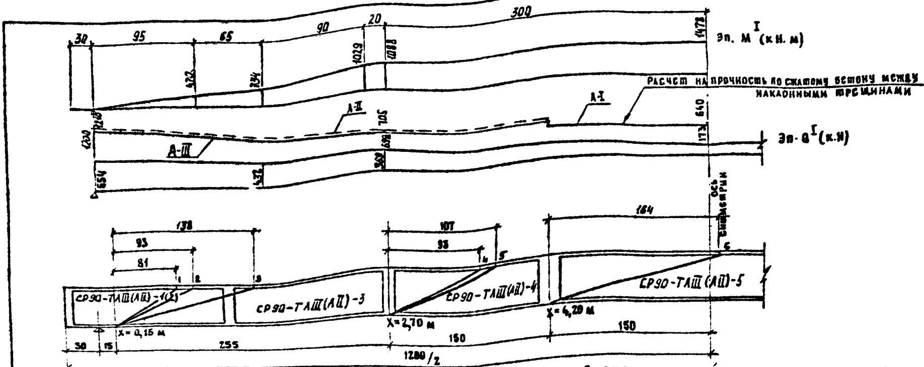
РАСЧЕТ СЕЧЕНИЙ, НАКАОННЫХ К ПРОДОЛЬНОЙ ОСИ ЭЛЕМЕНТА, НА ДЕЙСТВИЕ ИЗГИБАЮЩЕГО МОМЕНТА
